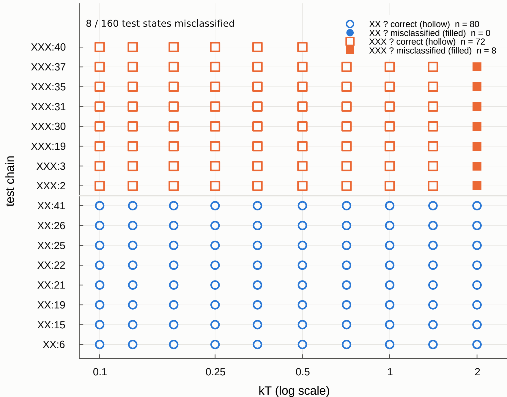
Alg 9 · classical ansatz + bias
