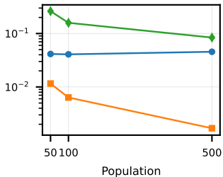
Griewank, D=10
