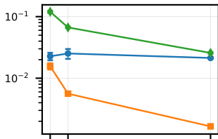
Griewank, D=10
