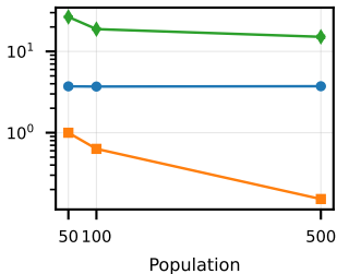
Griewank, D=100
