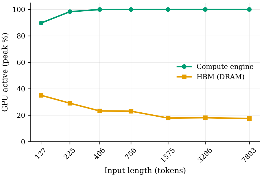
Prefill GPU utilisation — compute-bound
