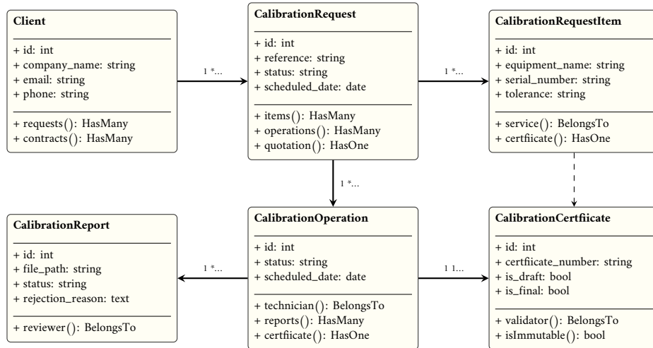
الشكل 3.7: مخطط فئات مجال المعايرة والمتروlogيا (Domain Class Diagram)
