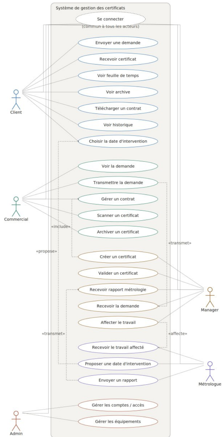
الشكل 3.1: المخطط العام لحالات الاستخدام لنظام إدارة الشهادات (Système de gestion des certificats)
