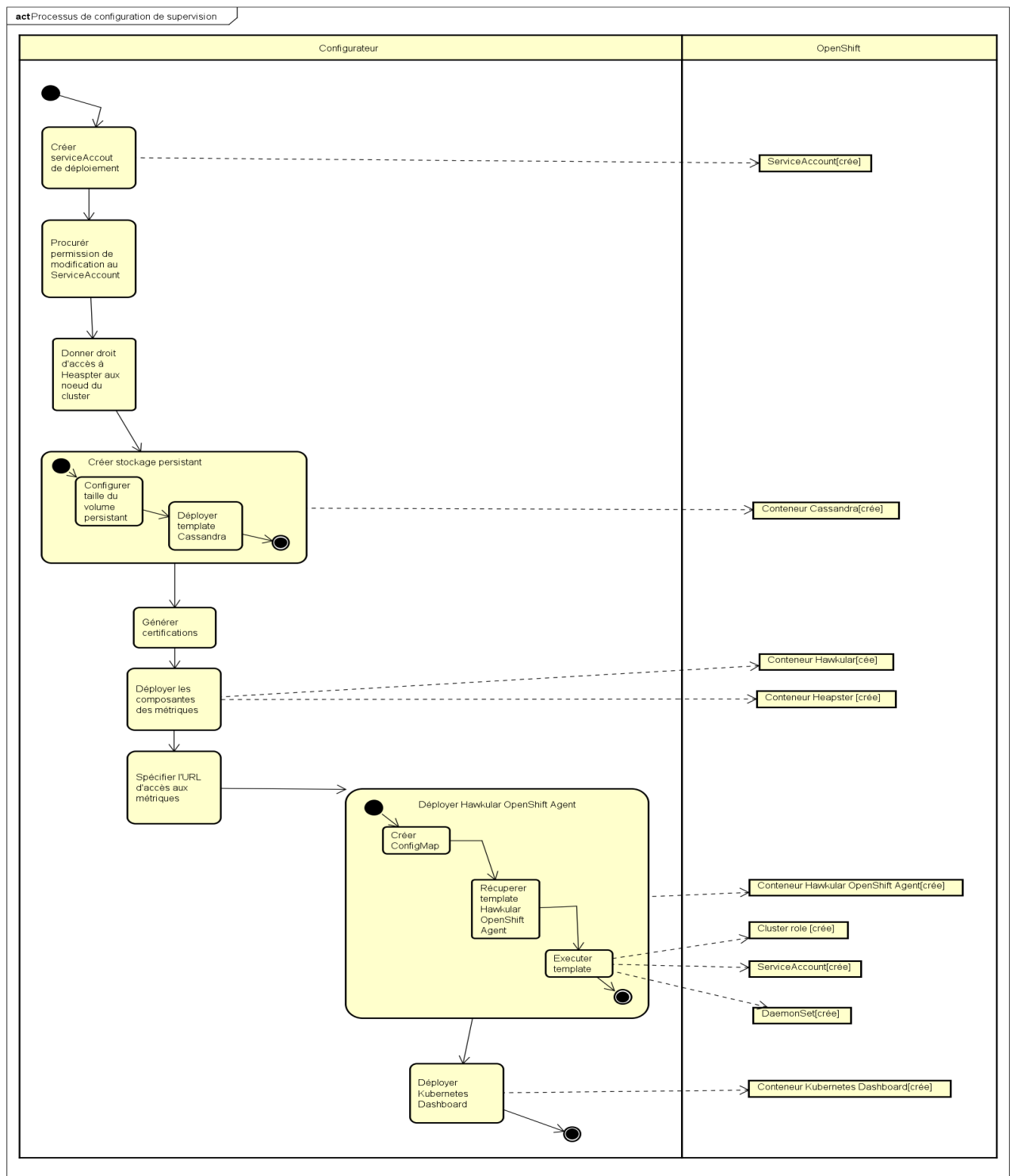
Figure 4.11: Processus de supervision de l'état du cluster
