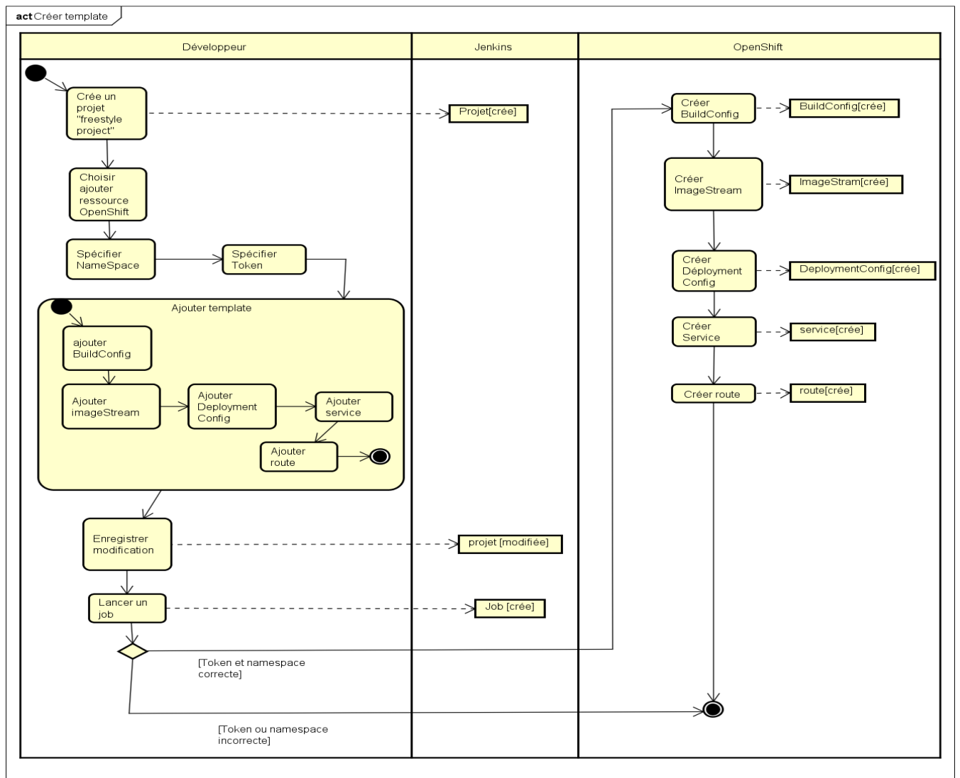
Figure 4.7: Processus de création d'un template
