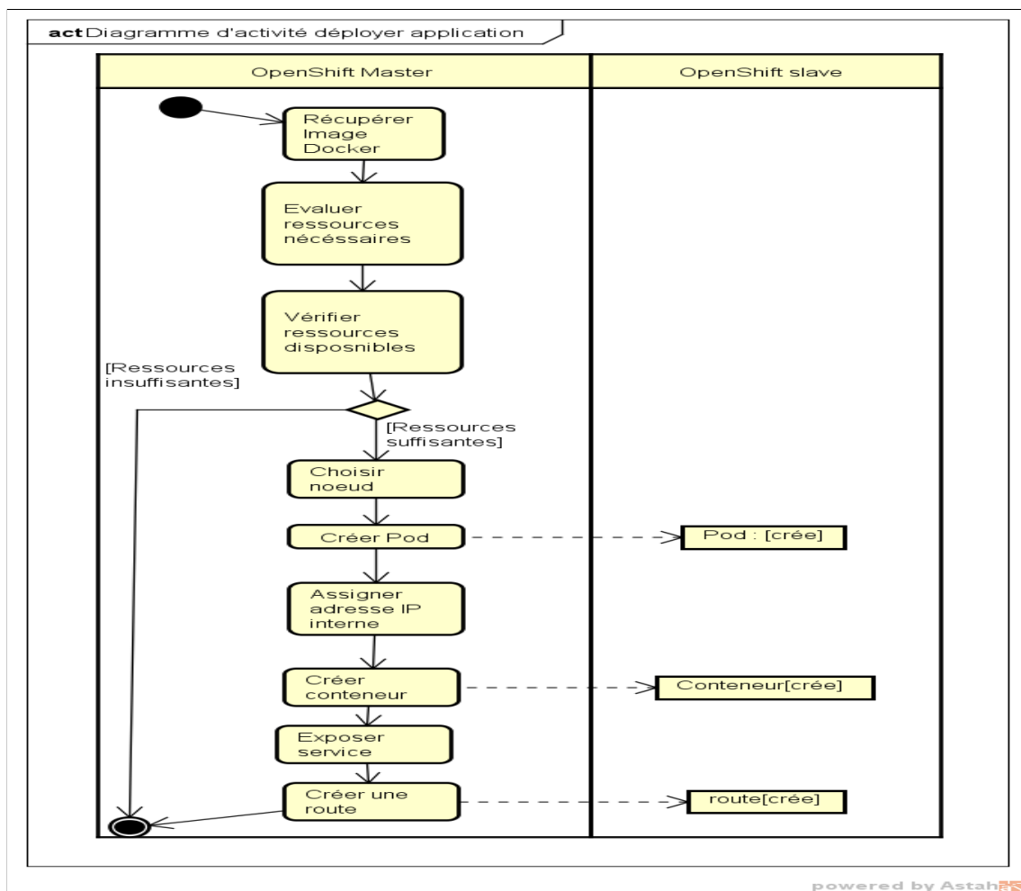
Figure 4.6: Processus de déploiement d'une application
