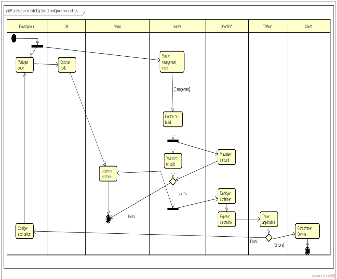
Figure 4.13: Processus d'intégration et de déploiement continu dans le pipeline
