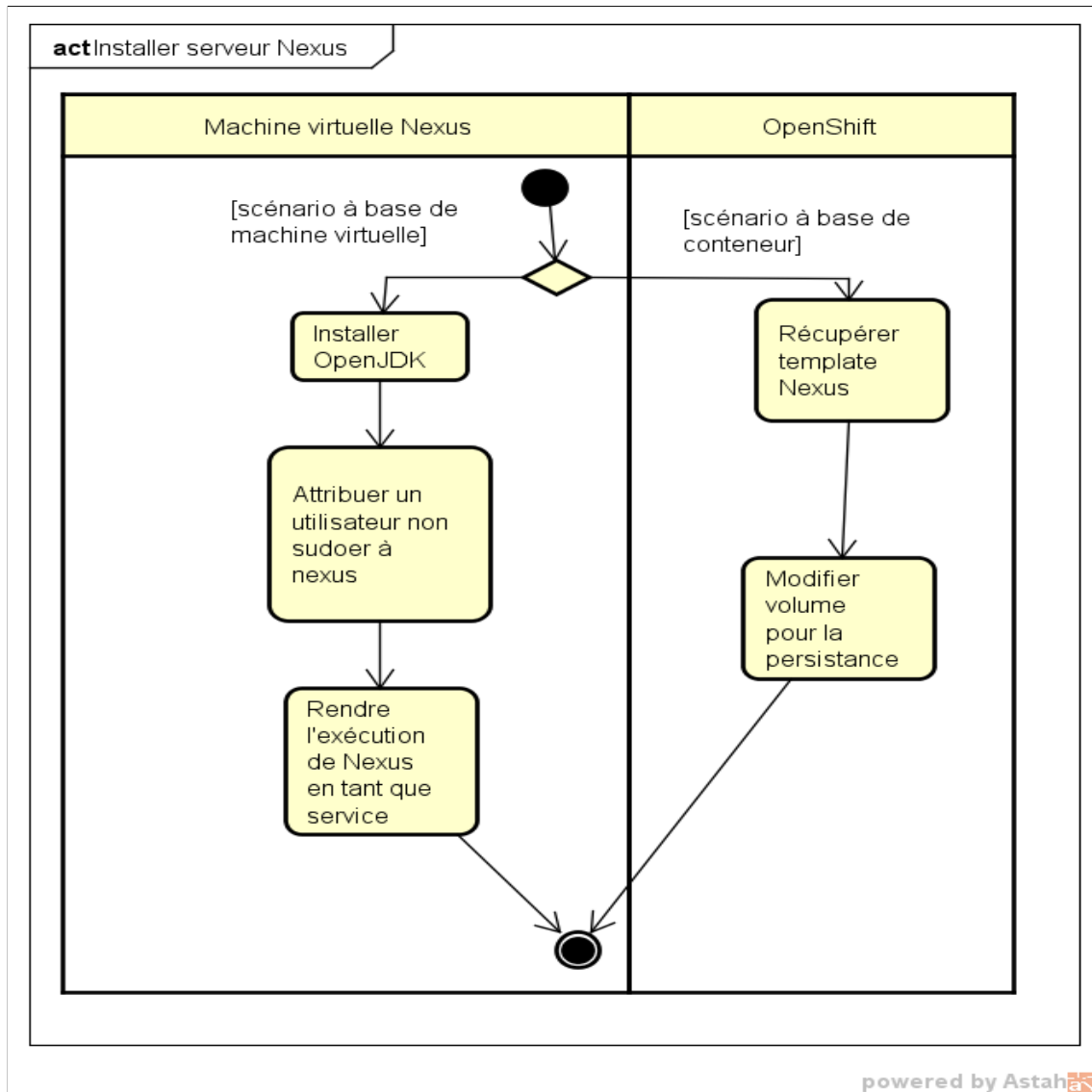
Figure 4.10: Processus d'installation du serveur Nexus
