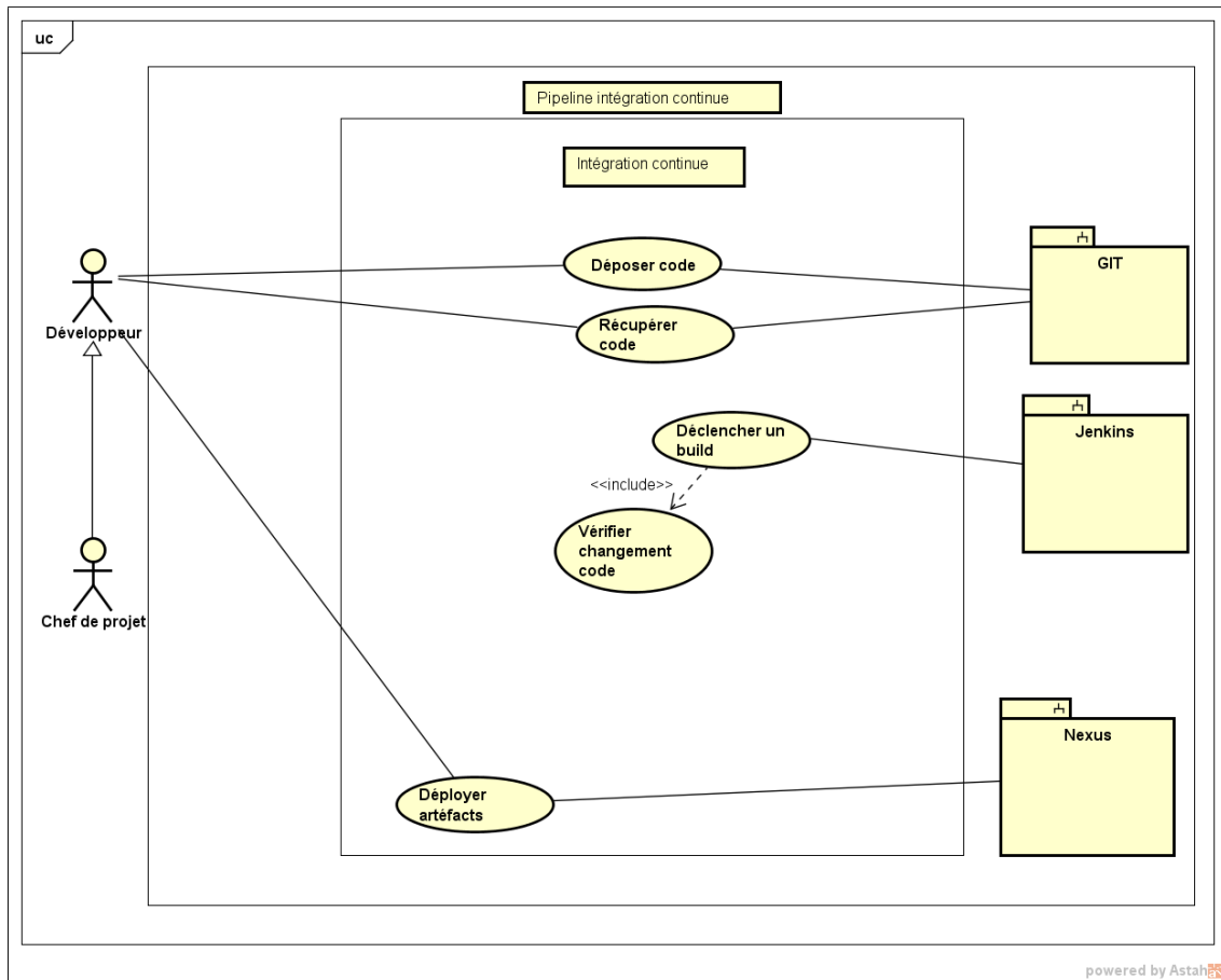
Figure 3.2: diagramme de cas d'utilisation "Intégration continue".
