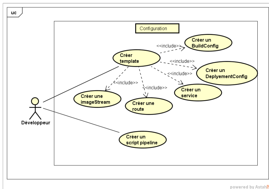
Figure 3.4: Diagramme de cas d'utilisation "Configuration".
