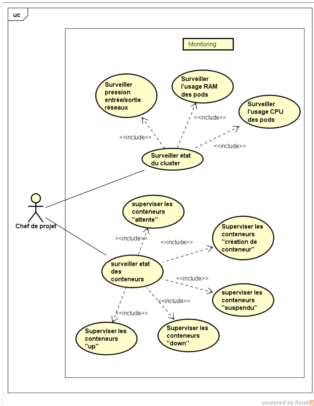
Figure 3.5: Diagramme de cas d'utilisation "Supervision".
