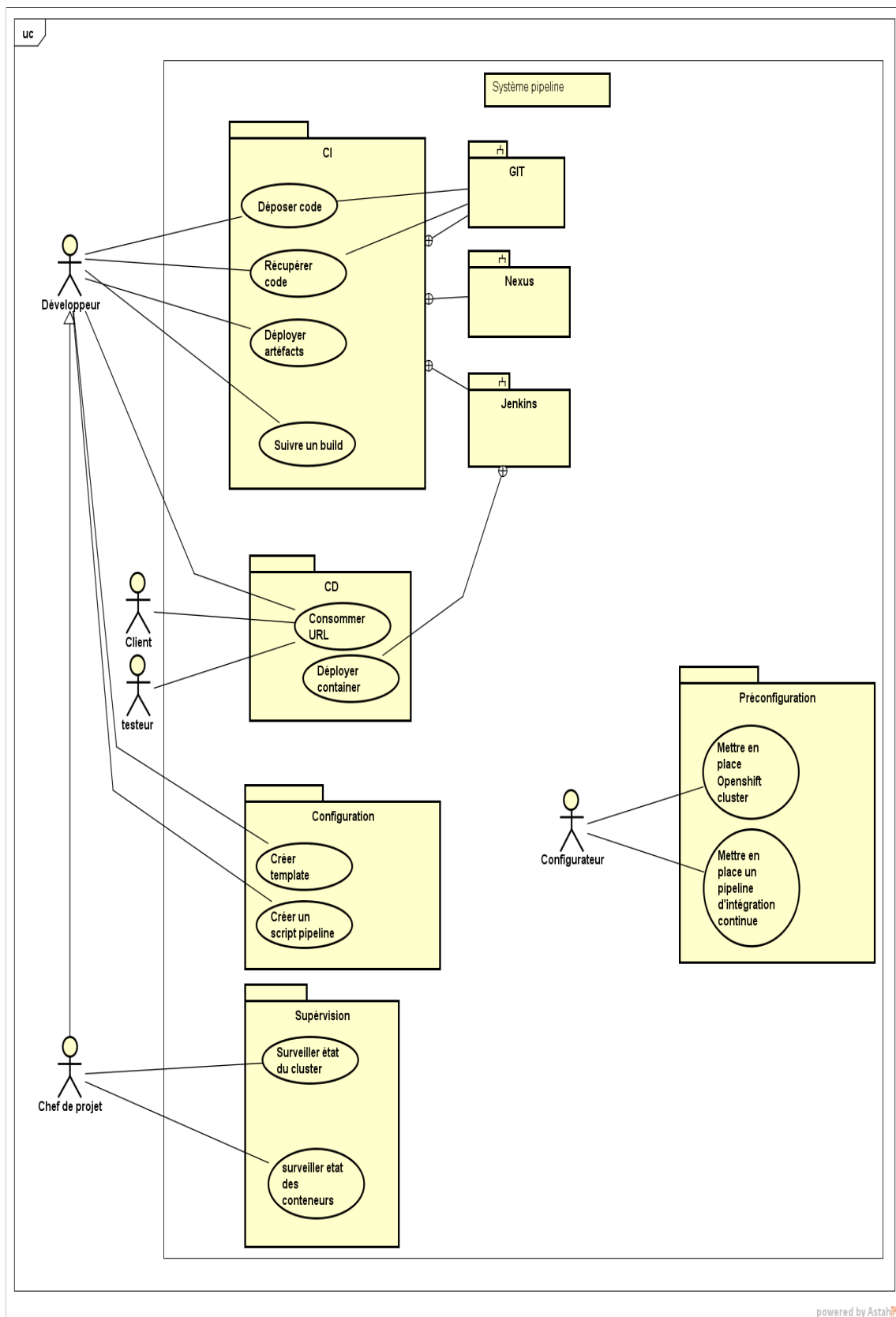
Figure 3.1: Diagramme de cas d'utilisation général.
