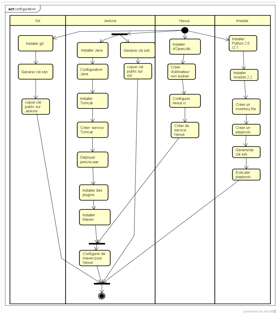
Figure 4.12: Processus pour la pré-configuration.
