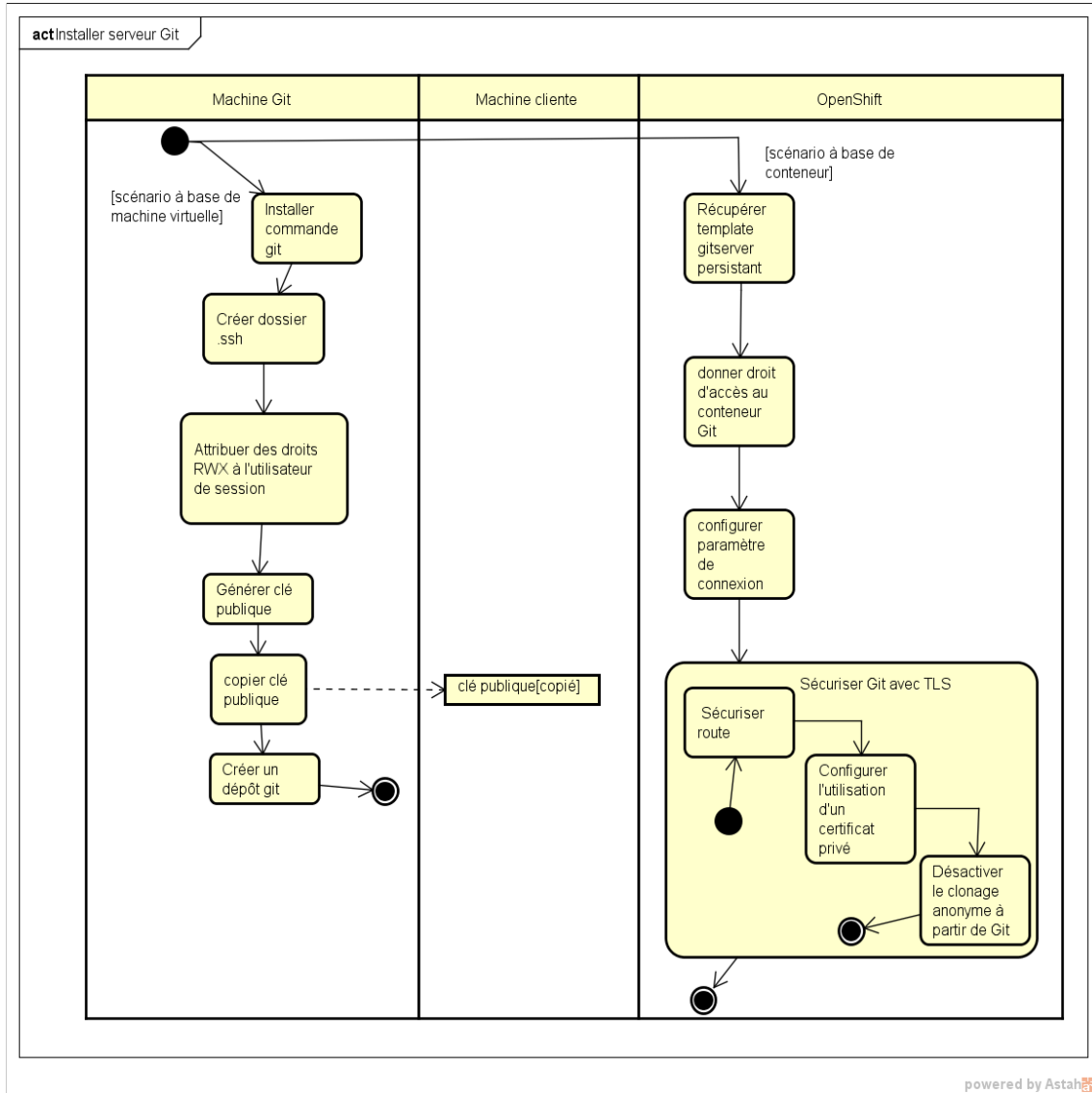
Figure 4.8: Processus d'installation du serveur Git
