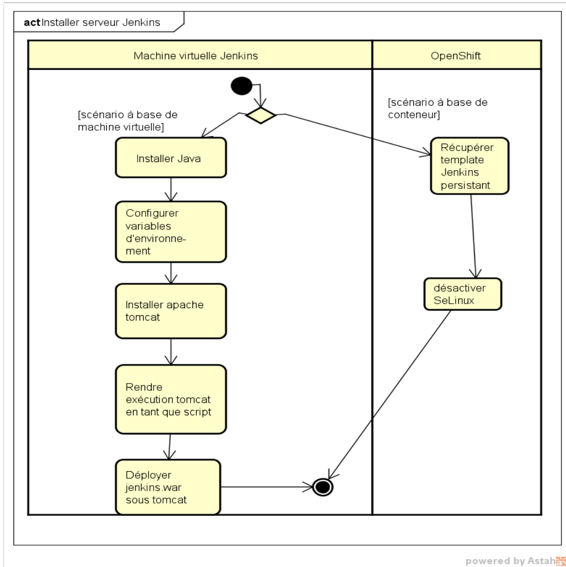
Figure 4.9: Processus d'installation du serveur Jenkins
