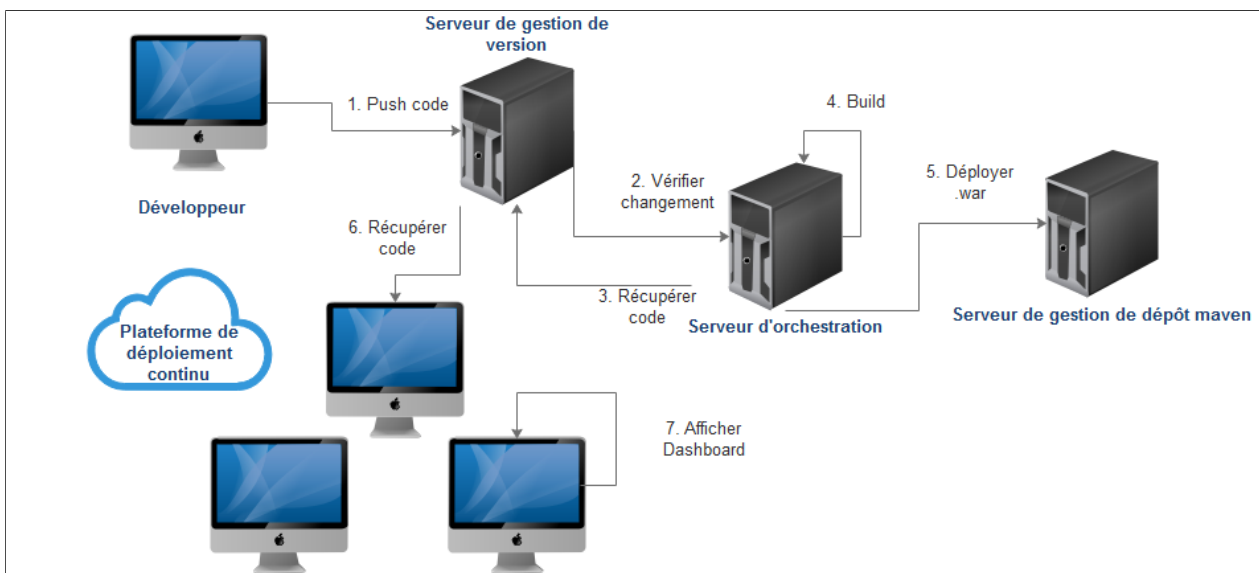
Figure 1.4: schéma explicatif de la solution proposée.
