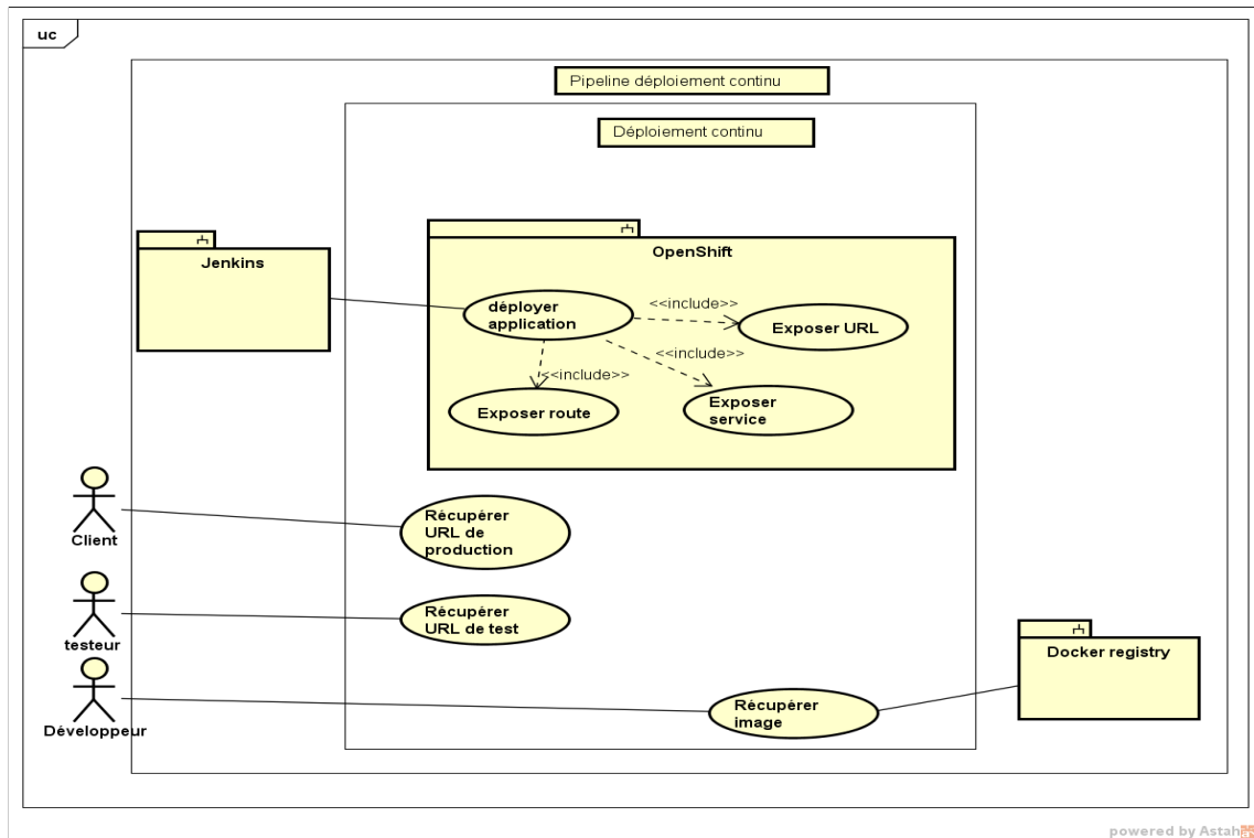
Figure 3.3: Diagramme de cas d'utilisation "Déploiement continu".
