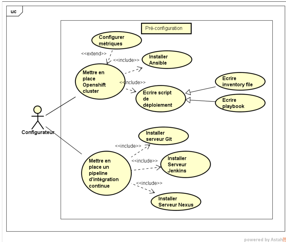
Figure 3.6: Diagramme de cas d'utilisation "Pré-configuration".
