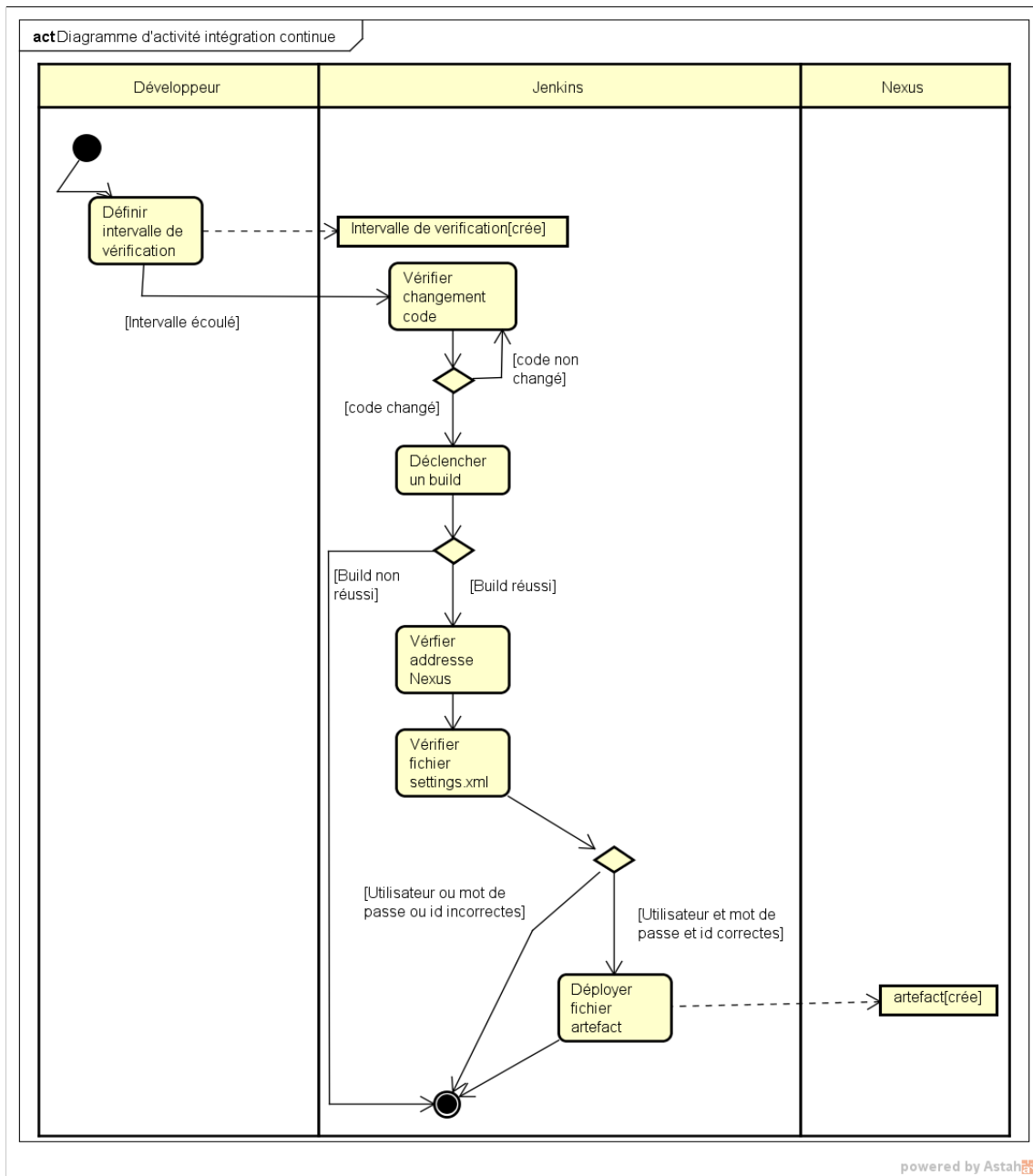
Figure 4.5: Processus d'Intégration continue
