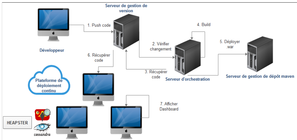
Figure 4.1: Schéma explicatif du pipeline intégration et déploiement continu.
