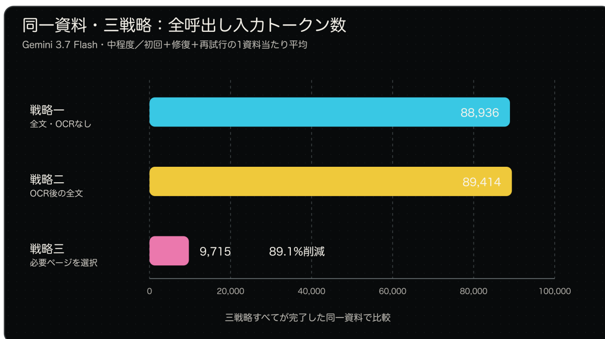
図5 三戦略の全呼出し入力トークン数
