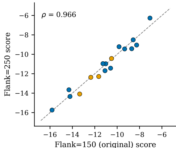
ESM-1b: flank=150 vs. flank=250
