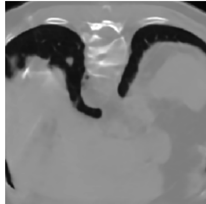
U-Net (large)
