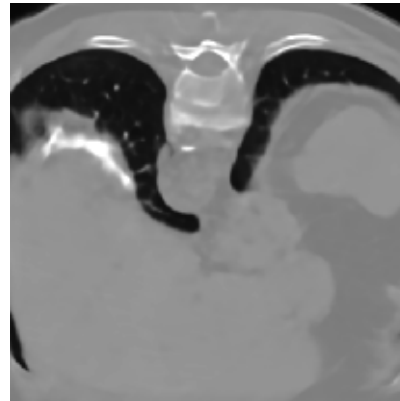
U-Net (large)
