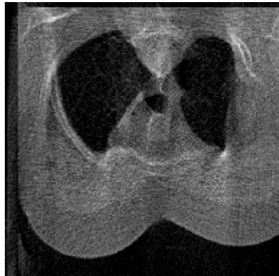
FBP (noisy)
