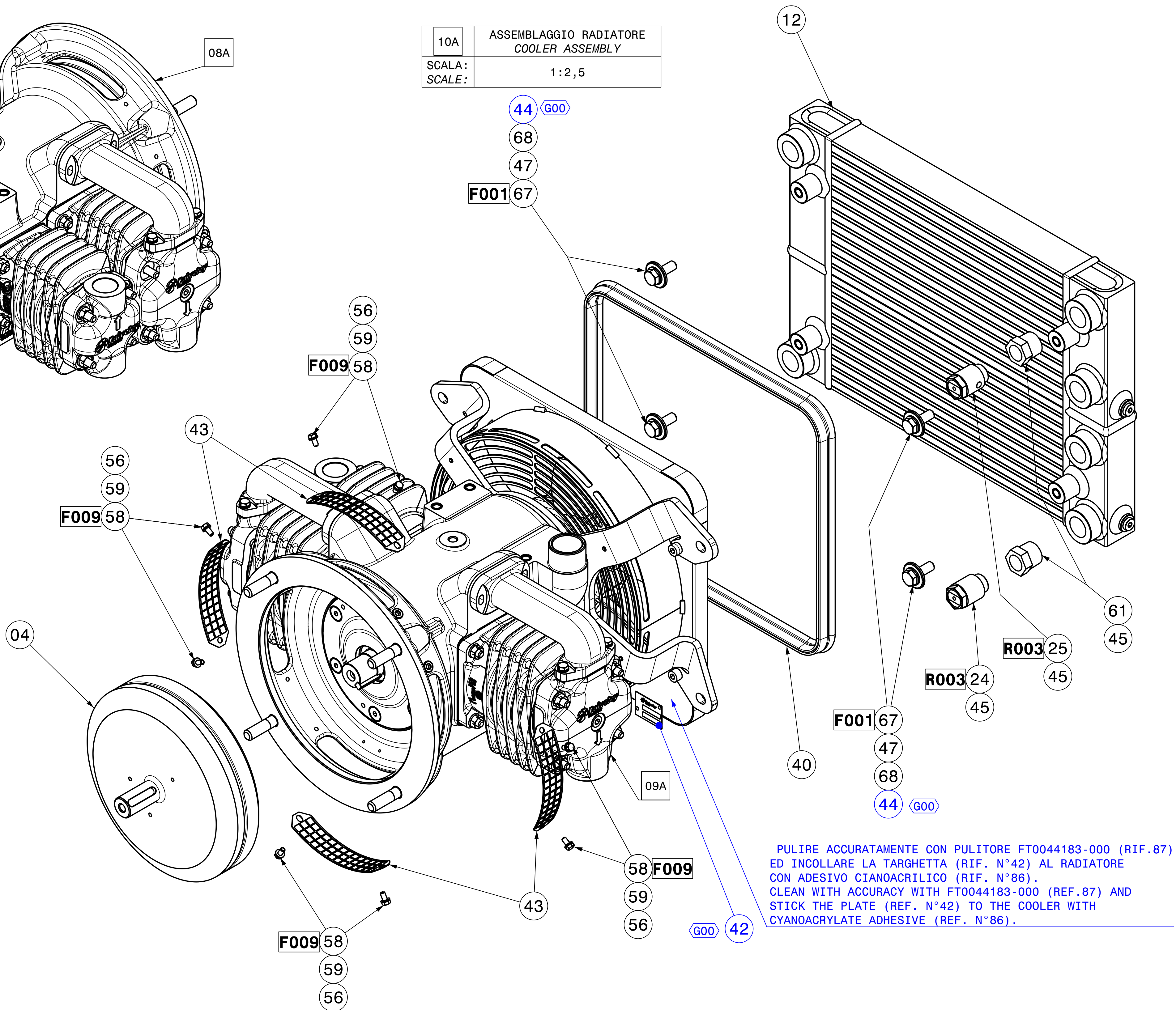
CONFIGURAZIONE STANDARD STANDARD CONFIGURATION FT0127469-100 1:2,5
