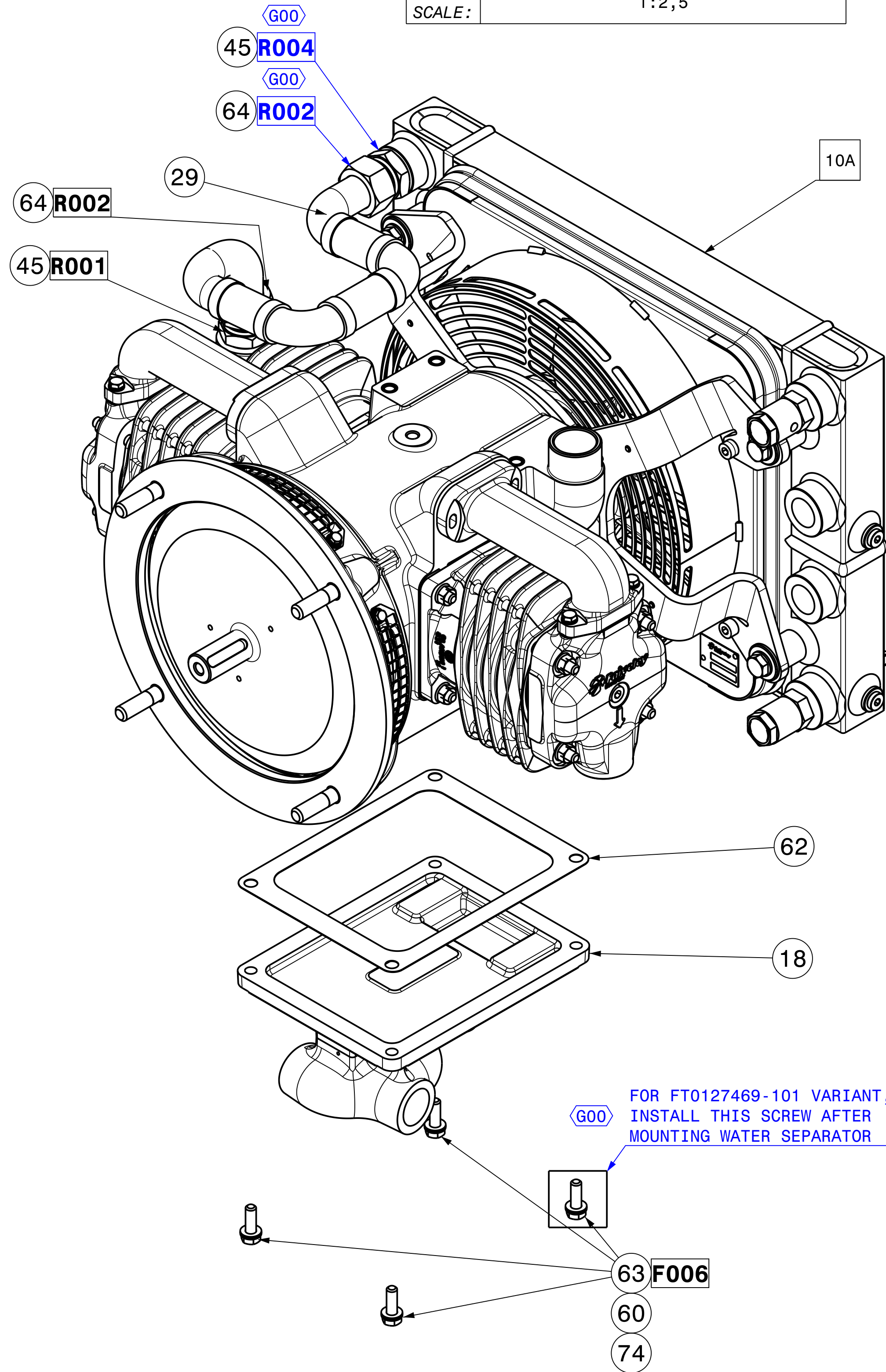
CONFIGURAZIONE ALTA' UMIDITA' HIGH HUMIDITY CONFIGURATION FT0127469-110 1:2,5
