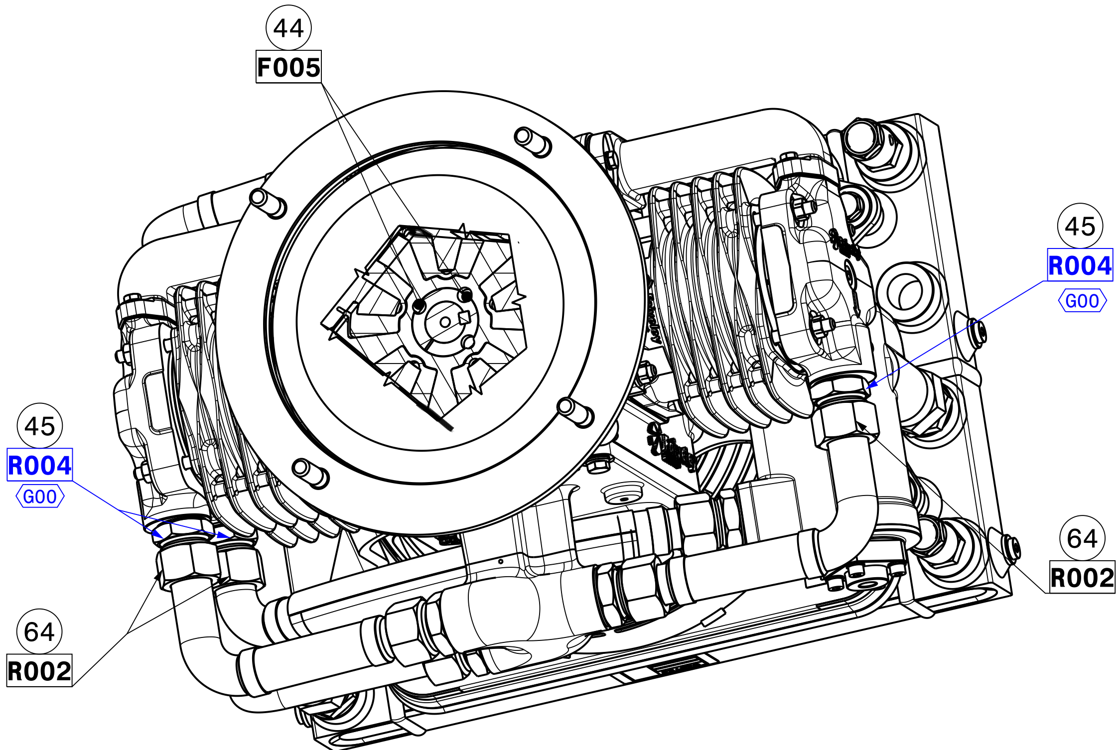
CONFIGURAZIONE ALTA' UMIDITA' HIGH HUMIDITY CONFIGURATION FT0127469-110 1:2,5
