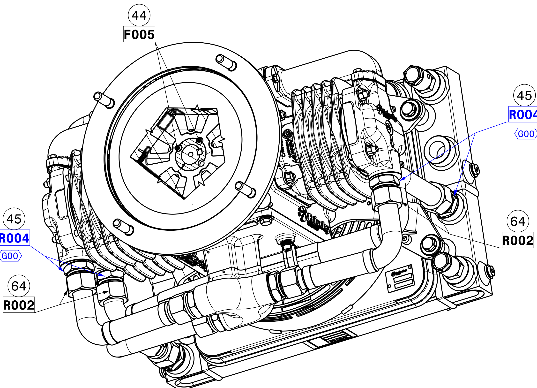
CONFIGURAZIONE STANDARD STANDARD CONFIGURATION FT0127469-100 1:2,5
