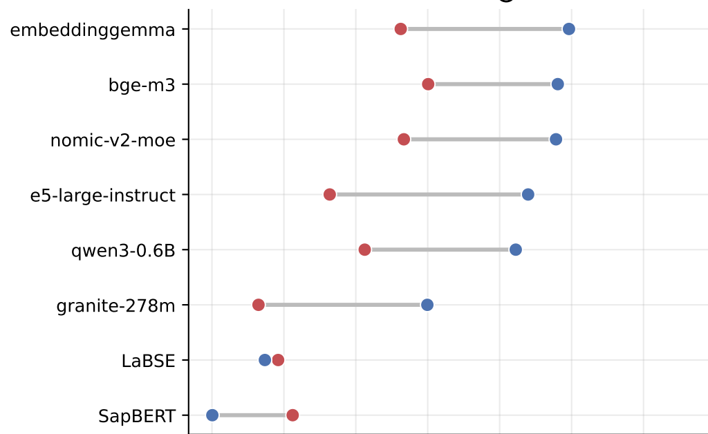
EPO — Hit@10
