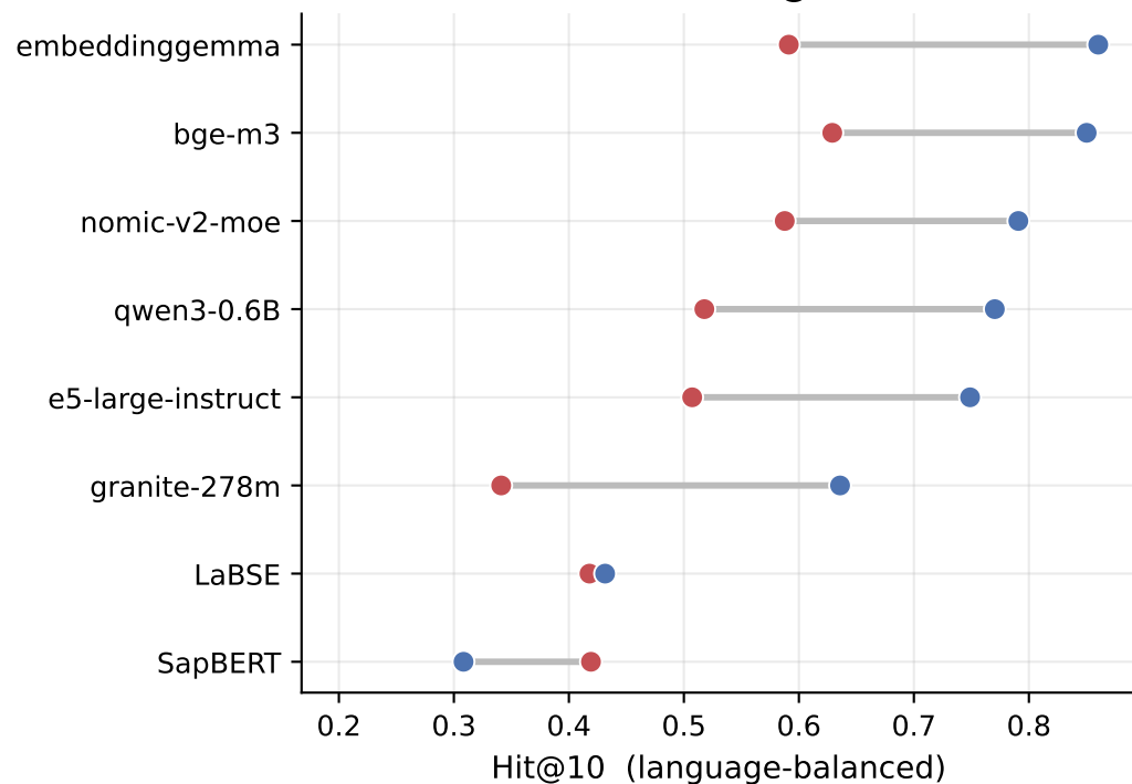
EPO — Hit@10
