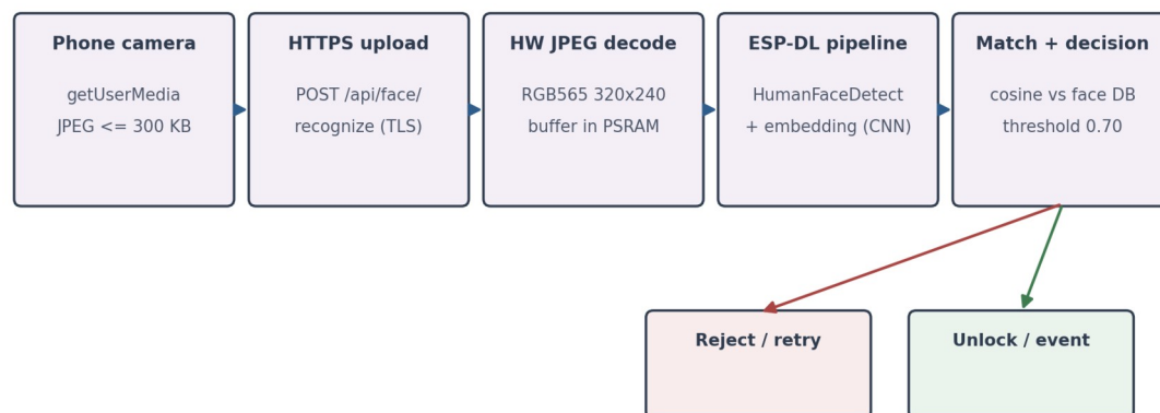
شکل ۶-۱: خط پردازش تشخیص چهره روی میکروکنترلر
