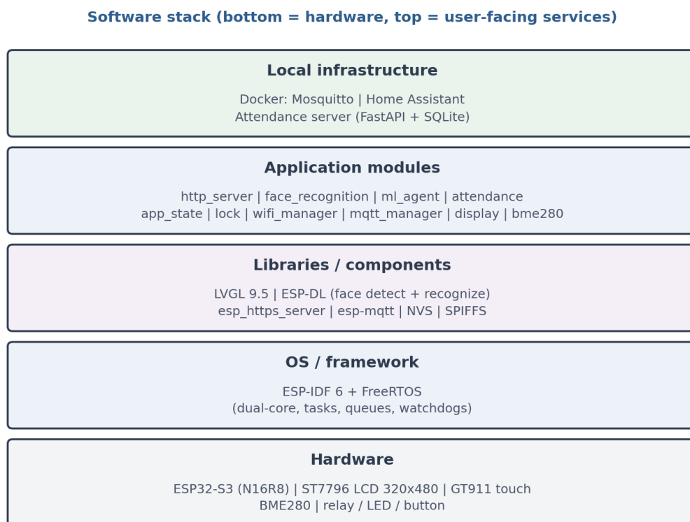
شکل ۴-۱: لایه‌های نرم‌افزاری سامانه
