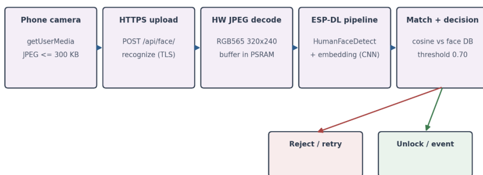
شکل ۶-۱: خط پردازش تشخیص چهره روی میکروکنترلر
