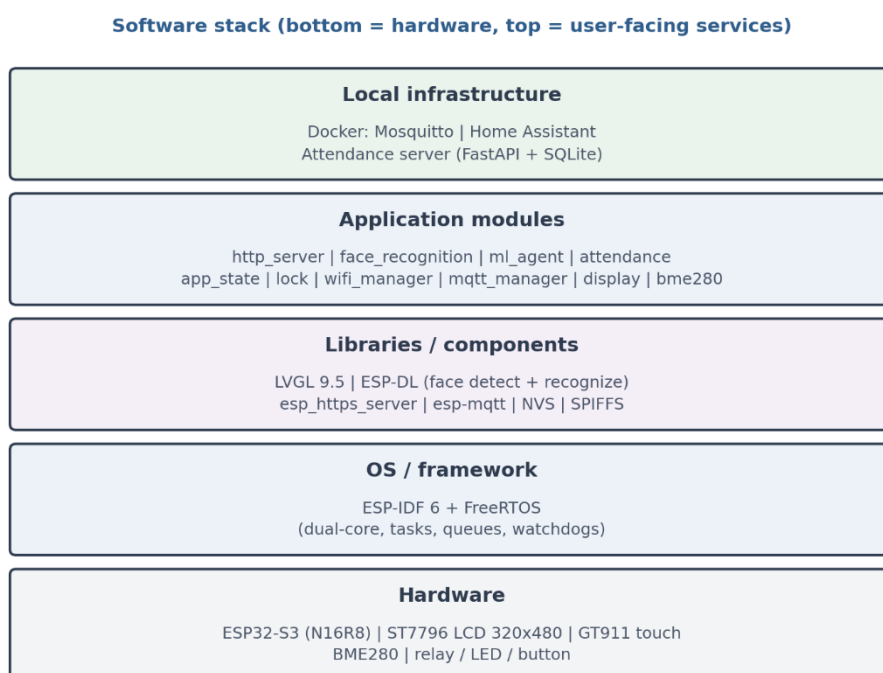
شکل ۴-۱: لایه‌های نرم‌افزاری سامانه
