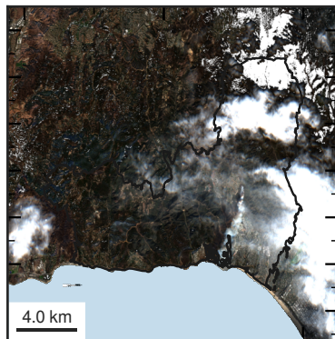
(b) True Color · Active fire
