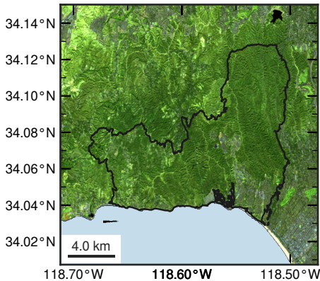
(d) False color · Pre-fire
