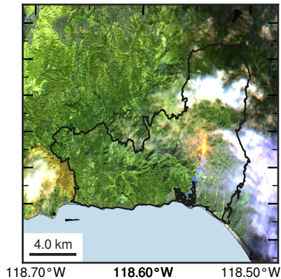
(e) False color · Active fire
