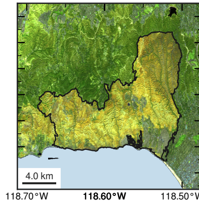
(f) False color · Post-fire
