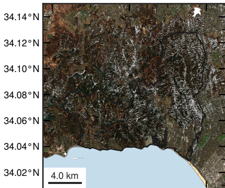
(a) True Color · Pre-fire
