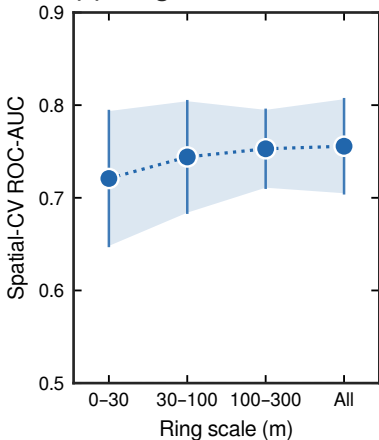
(a) Ring-scale AUC
