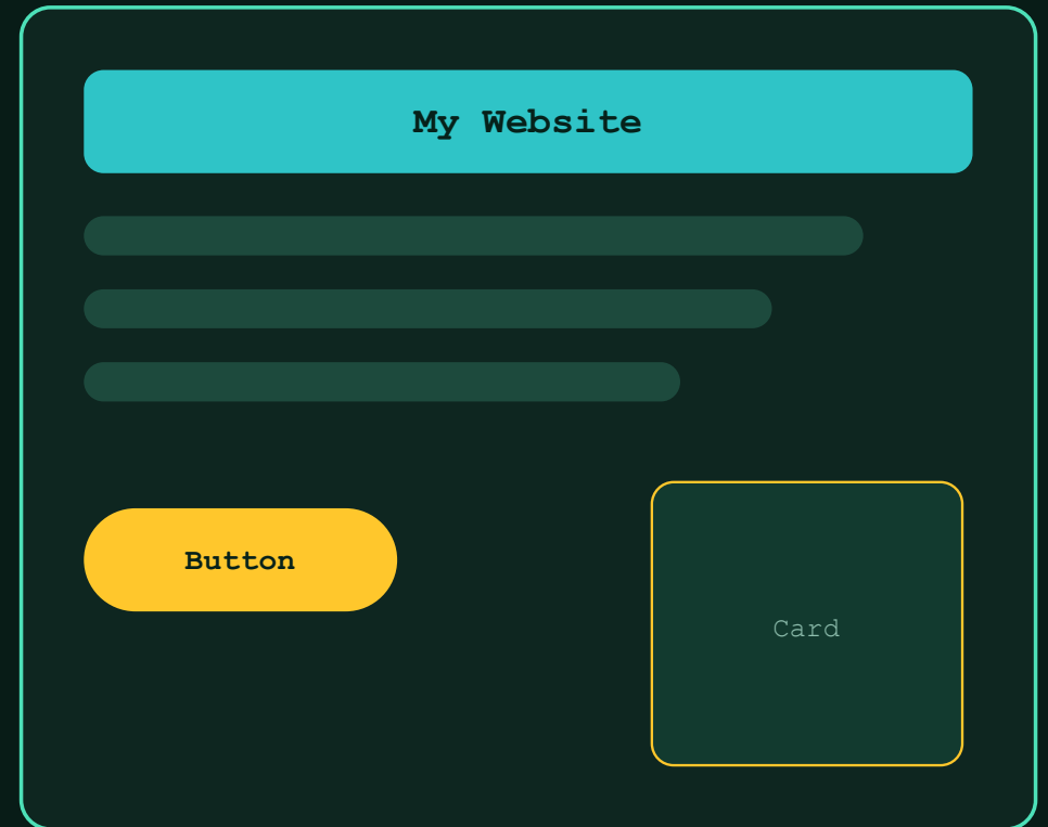
HTML + CSS
