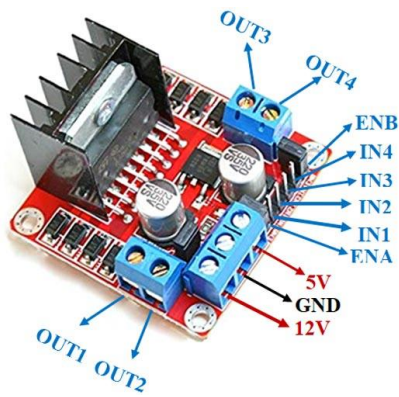
FIG 2.4.1 L298N Module PINS
