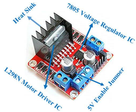
FIG 2.4.2 L298N Module
