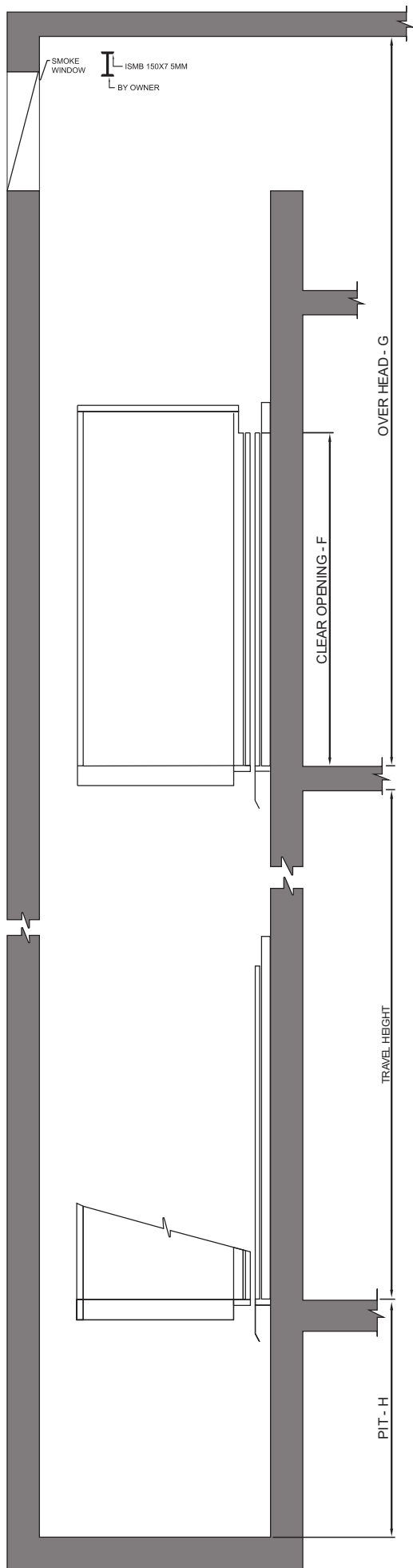
HOISTWAY ELEVATION
