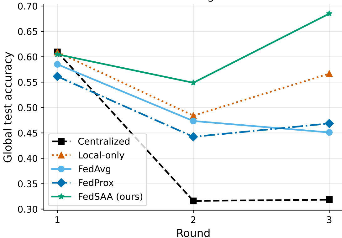
F1: Convergence
