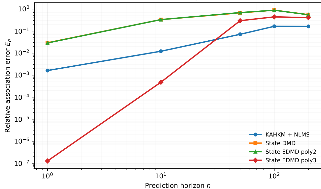
Van der Pol external Koopman baselines
