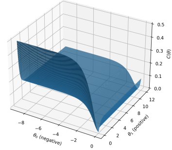
Fig. 4: C(\theta)
