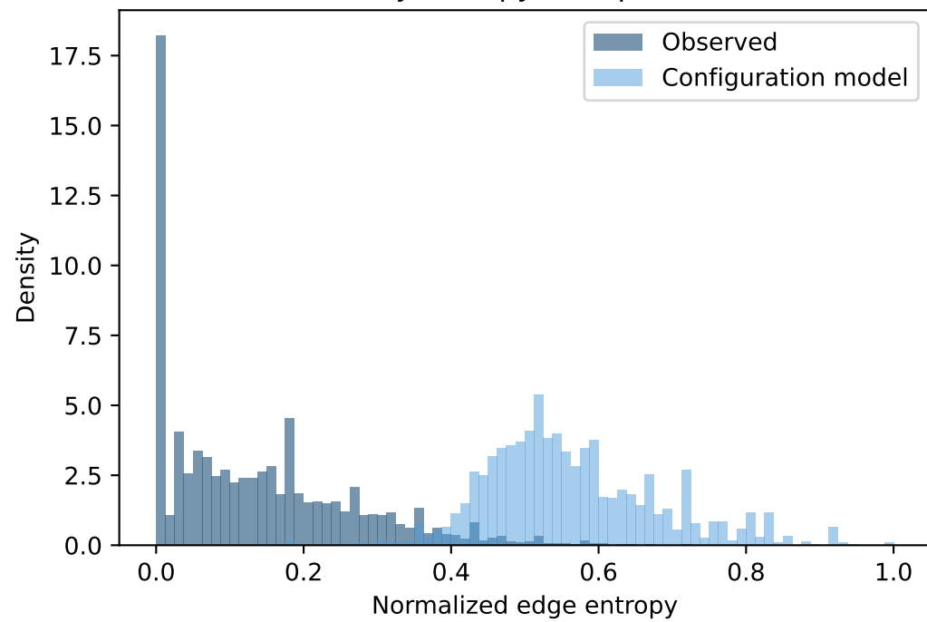
(d) Community entropy (independent Leiden)
