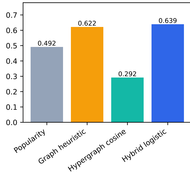
Hit@10
