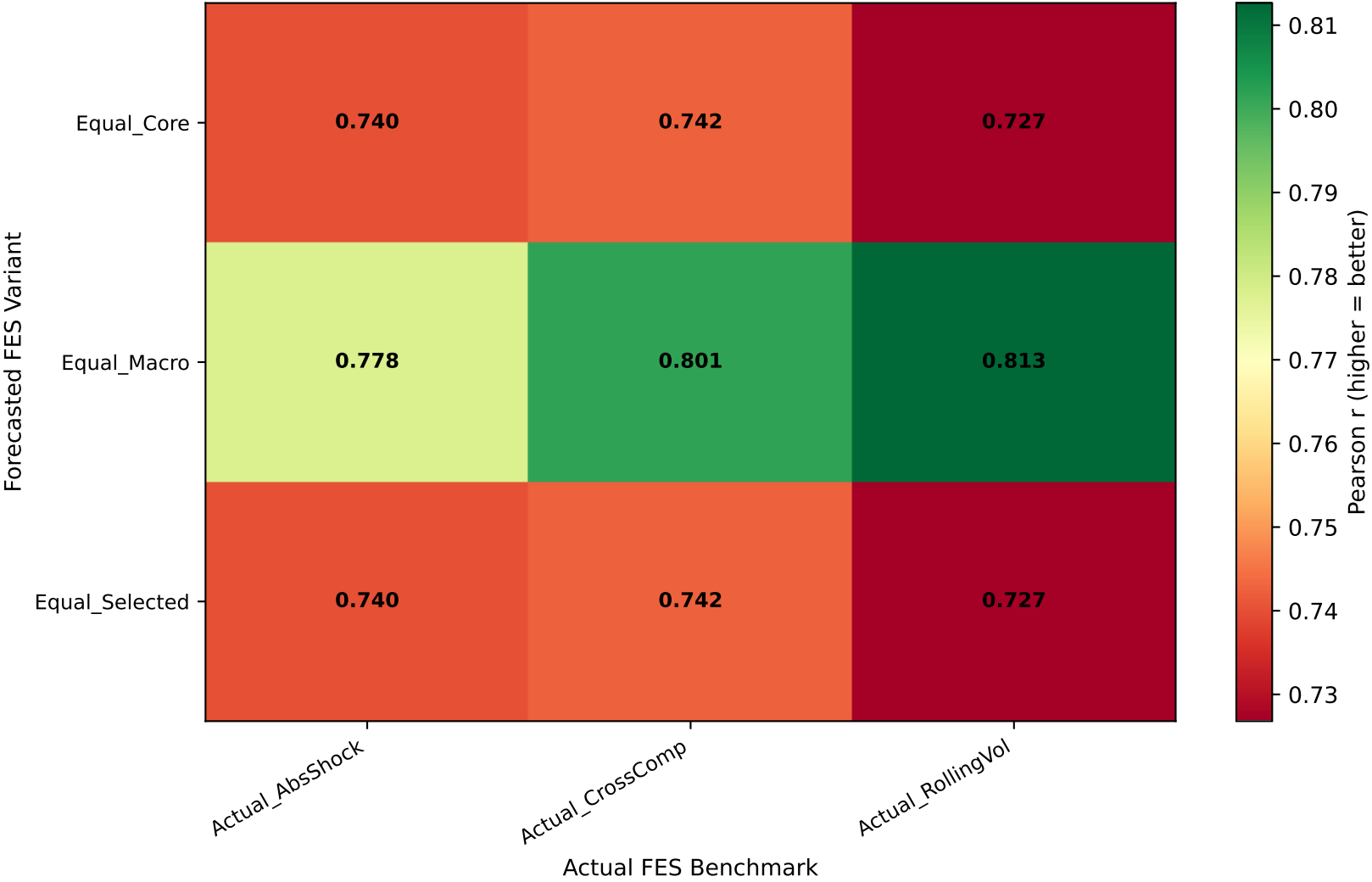
FES Robustness — Pearson_r: Forecasted vs Actual Benchmarks
