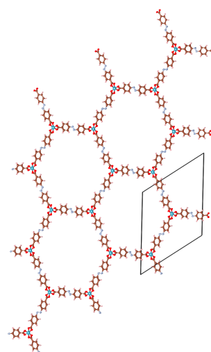
qmof-52ef7e9
