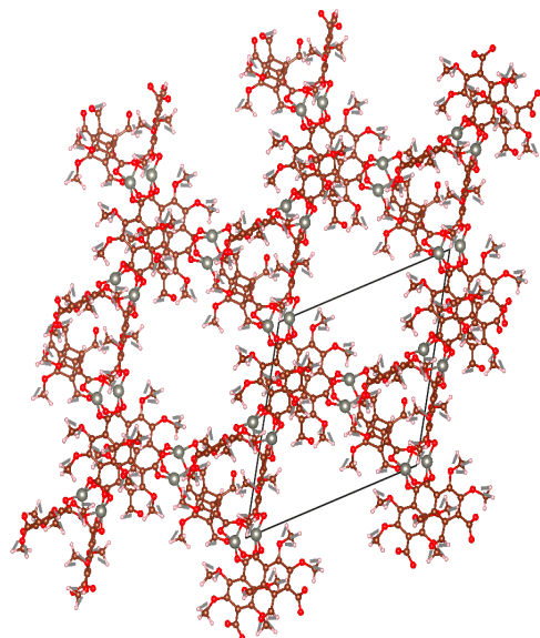
qmof-07c07d3
