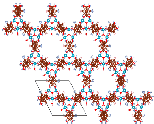
qmof-91692c9
