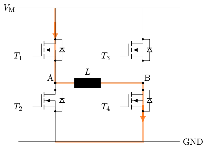
Abbildung 2.8: Aufbau einer H-Brücke aus zwei Halbbrückenzeigen. Die Wicklung liegt als Diagonale zwischen den Mittelpunkten A und B. Hervorgehoben ist der Strompfad bei durchgeschaltetem T_1 und T_4 ; das Durchschalten von T_2 und T_3 kehrt die Stromrichtung um.
