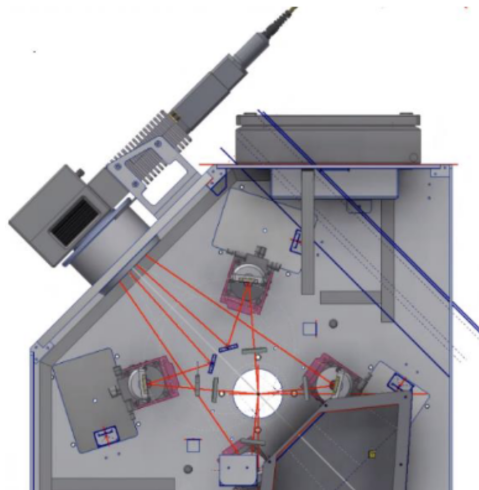
Abbildung 3.3: wireLINE MIRROR System - Laserstrahlführung, CleanLaser2022
