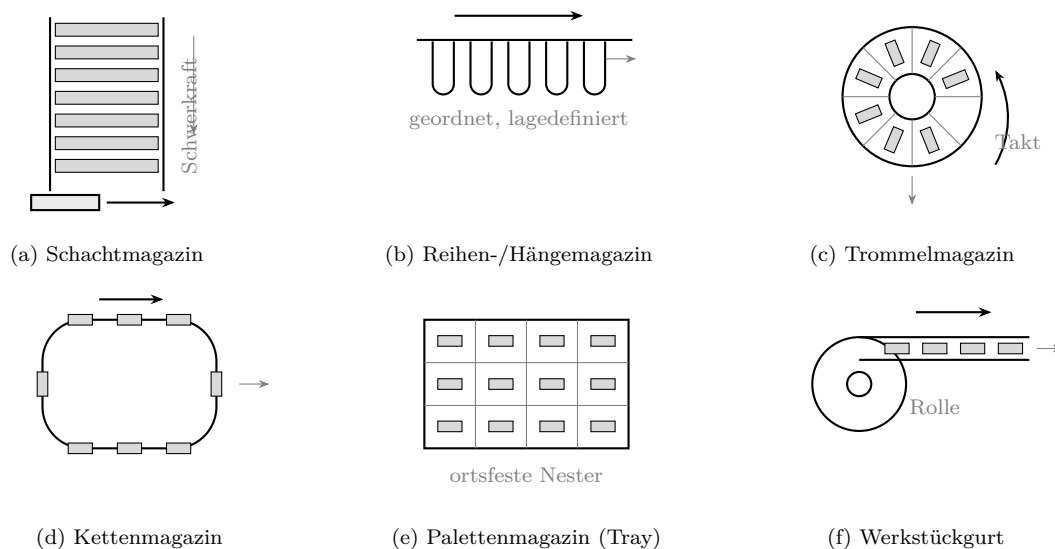
Abbildung 3.5: Bauformen geordneter Magazine zur lagedefinierten Bevorratung von Werkstücken. Eigene Darstellung in Anlehnung an GrundlagenHandhabungstechnik.2020 .
