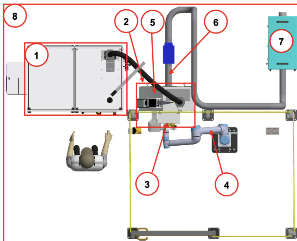
Abbildung 3.1: Gesamtansicht des Laserbearbeitungssystems, CleanLaser2022
