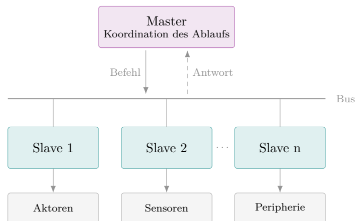
Abbildung 2.6: Aufbau in einer Master-Slave-Architektur.
