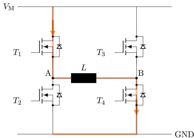
Abbildung 2.7: Aufbau einer H-Brücke aus zwei Halbbrücken zweigen. Die Wicklung liegt als Diagonale zwischen den Mittelpunkten A und B. Hervorgehoben ist der Strompfad bei durchgeschaltetem T_1 und T_4 ; das Durchschalten von T_2 und T_3 kehrt die Stromrichtung um.
