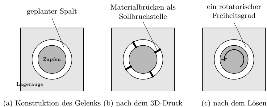
Abbildung 5.1: Schematische Schnittdarstellung eines im Druckprozess erzeugten Gelenks: (a) Zapfen und Lagerauge werden mit einem geplanten Spalt als ein Bauteil modelliert, (b) beim Druck verbleiben Materialbrücken als Sollbruchstelle, (c) nach dem Lösen und Austragen der Materialbrücken durch wiederholtes Bewegen verbleibt ein rotatorischer Freiheitsgrad.
