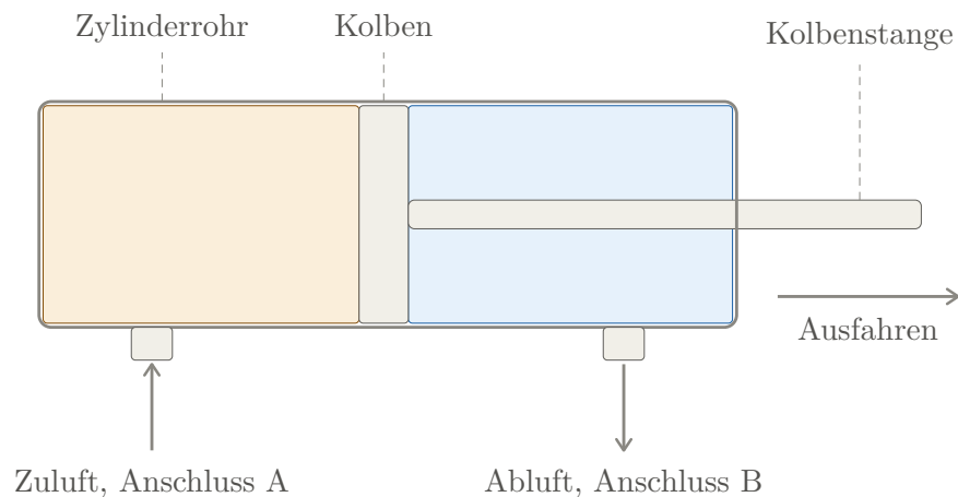
Abbildung 2.2: Schnittzeichnung eines doppelwirkenden Pneumatikzylinders
