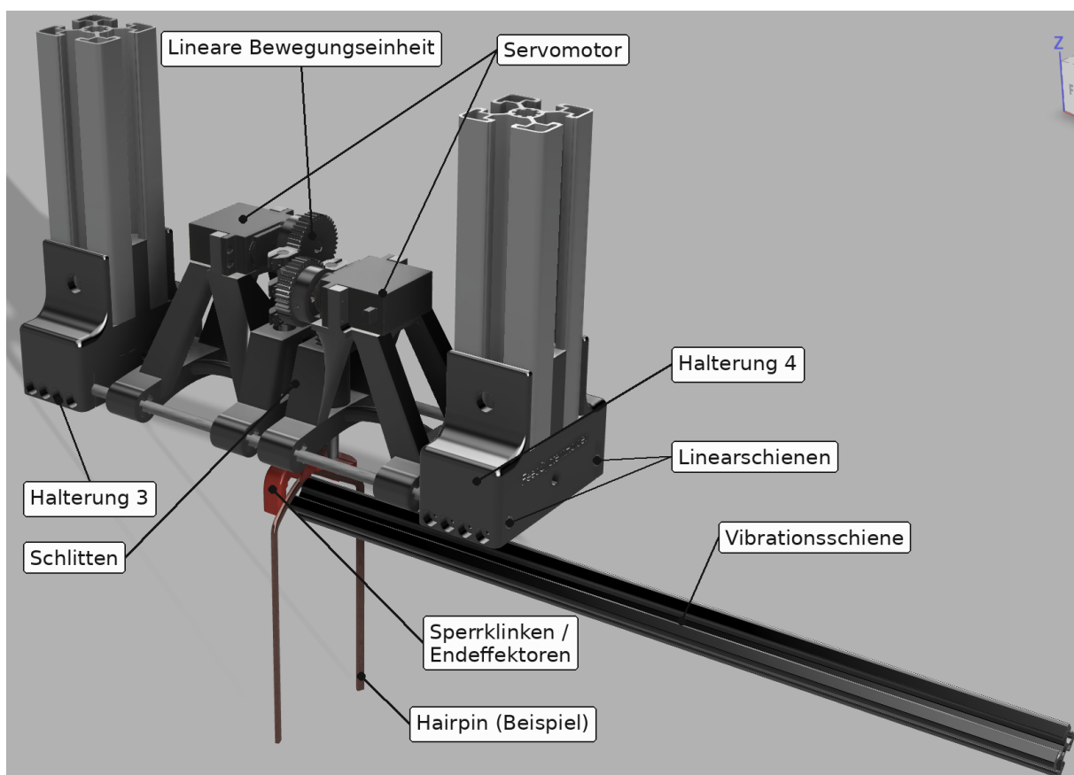
Abbildung 5.3: Aufbau der Vereinzelungseinheit
