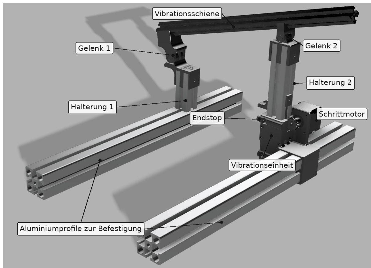
Abbildung 5.2: Aufbau der Vibrationsschiene
