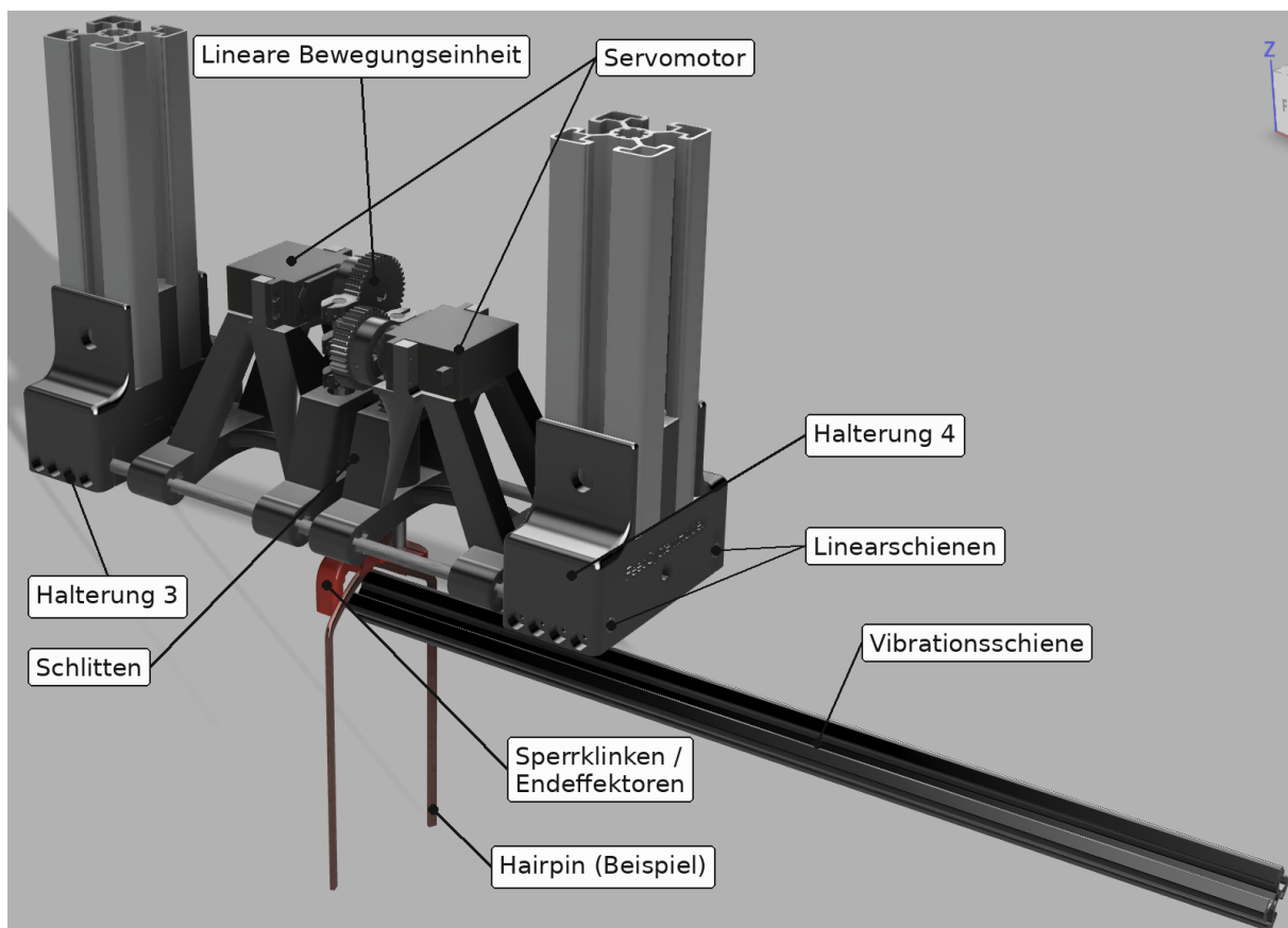
Abbildung 5.3: Aufbau der Vereinzelnungseinheit
