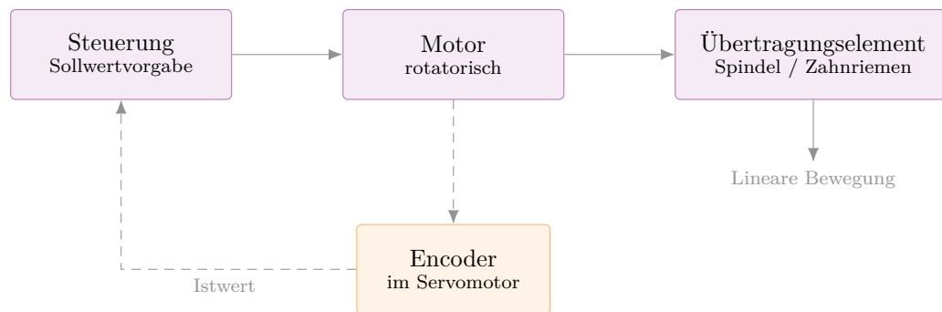
Abbildung 2.3: Wirkkette eines Servontriebs mit integriertem Regelkreis zur Lagerückführung.
