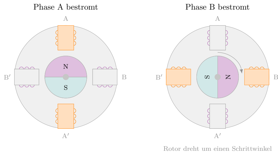
Abbildung 2.3: Funktionsprinzip des zweiphasigen Schrittmotors. Das Weiterschalten der Bestromung von Phase A auf Phase B dreht den Rotor um einen Schrittinkel. Stark vereinfachte Darstellung mit vier Statorpolen; reale Hybrid-Schrittmotoren erreichen durch Rotorbezahnung Schrittinkel von typischerweise 1,8^\circ .
