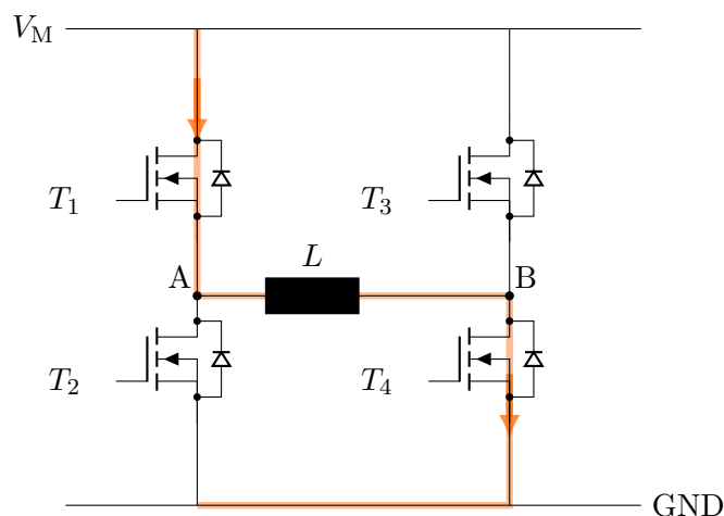
Abbildung 2.8: Aufbau einer H-Brücke aus zwei Halbbrücken. Die Wicklung liegt als Diagonale zwischen den Mittelpunkten A und B. Hervorgehoben ist der Strompfad bei durchgeschaltetem T_1 und T_4 ; das Durchschalten von T_2 und T_3 kehrt die Stromrichtung um.
