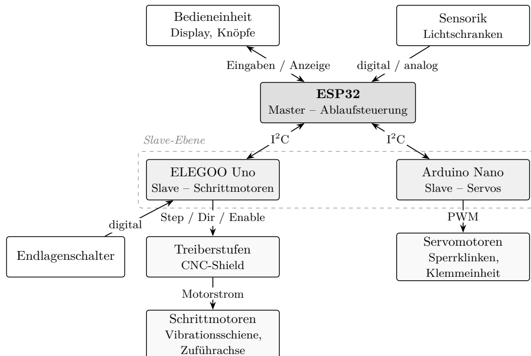
Abbildung 5.6: Signalfluss Diagramm
