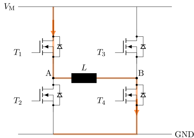
Abbildung 2.7: Aufbau einer H-Brücke aus zwei Halbbrückenzeigen. Die Wicklung liegt als Diagonale zwischen den Mittelpunkten A und B. Hervorgehoben ist der Strompfad bei durchgeschaltetem T_1 und T_4 ; das Durchschalten von T_2 und T_3 kehrt die Stromrichtung um.
