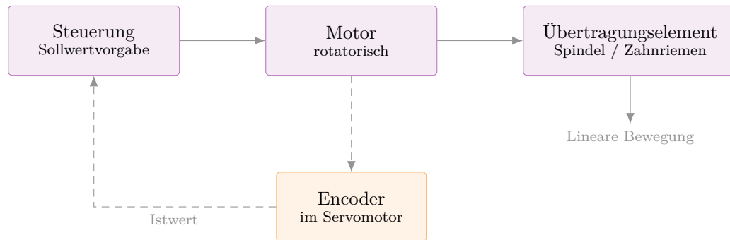
Abbildung 2.3: Wirkkette eines Servontriebs mit integrierem Regelkreis zur Lagerückführung.
