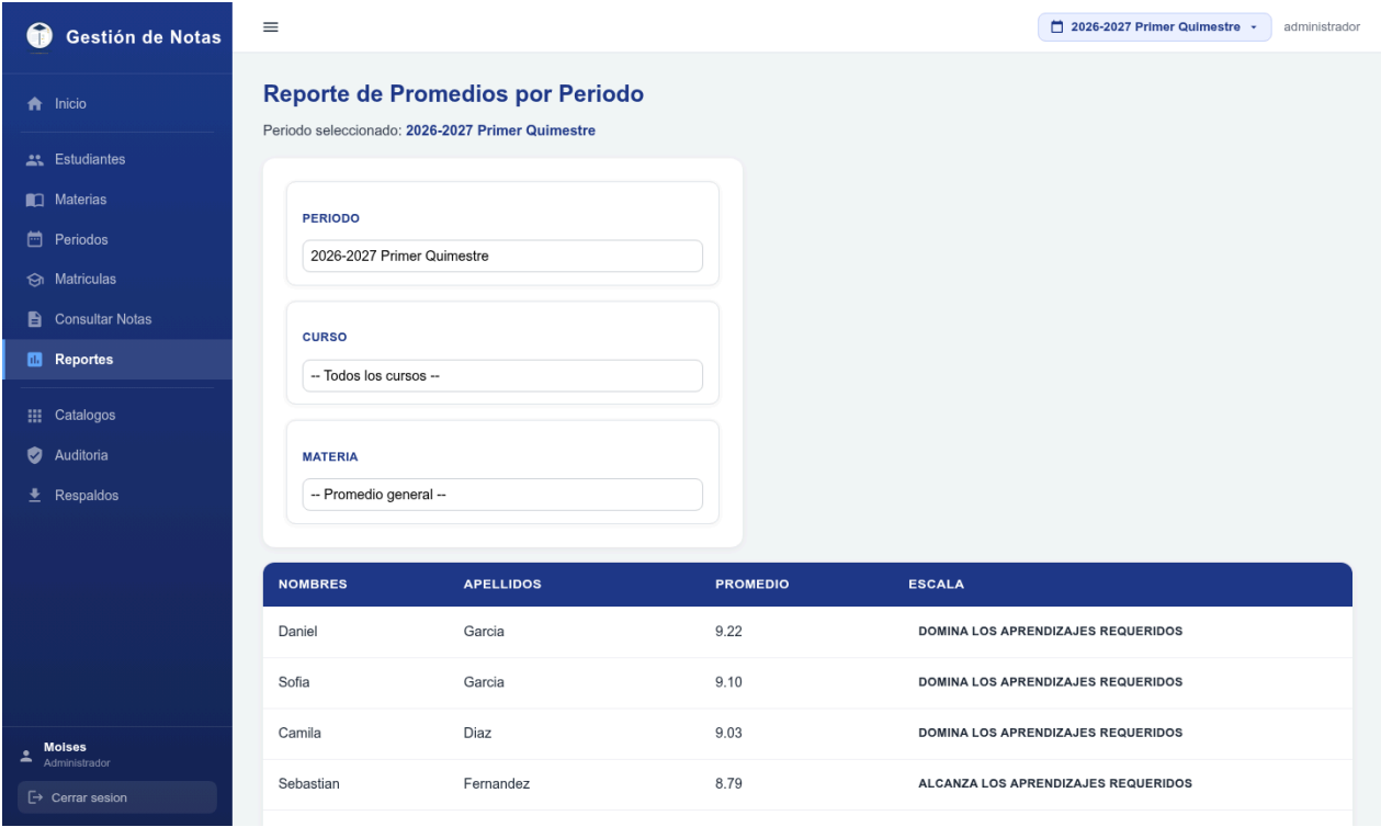
Figura 26. Reporte de promedios (UAT-05).
