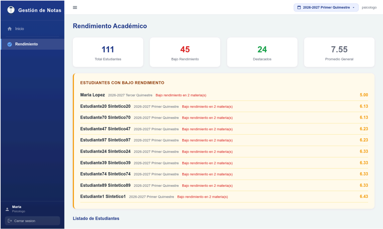
Figura 28. Panel de rendimiento de la psicóloga (UAT-07).
