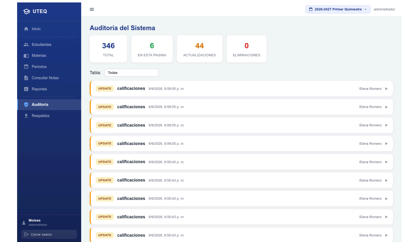
Figura 11. Panel de auditoría del administrador ('playwright-03-admin-auditoria.png').
