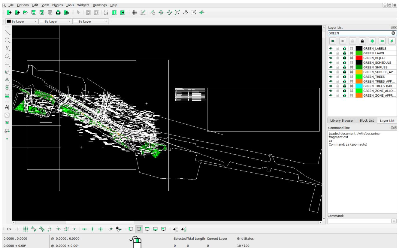
Рис. 5.2. Тот же чертёж, список слоёв с фильтром GREEN: 11 слоёв результата отдельно от исходных, каждый включается и выключается сам по себе.
