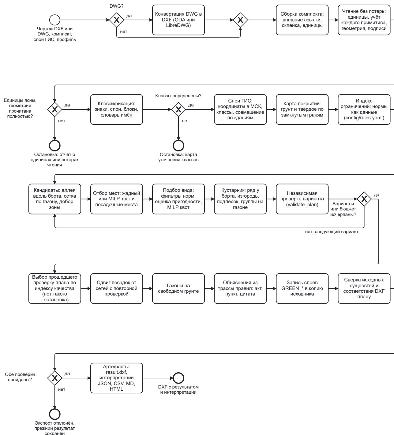
Рис. 3.1. Прогон: от входного чертежа до выходного DXF и интерпретаций. Шлюзы проверок входа и выхода с исходом «нет» заканчиваются остановкой с отчётом, а не допусанием; шлюз портфеля с исходом «нет» переходит к следующему варианту.
