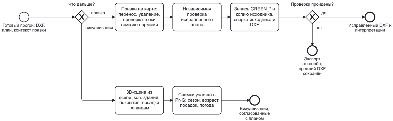
Рис. 3.2. После прогона: правка на карте с пересборкой DXF и 3D-визуализация участка.
