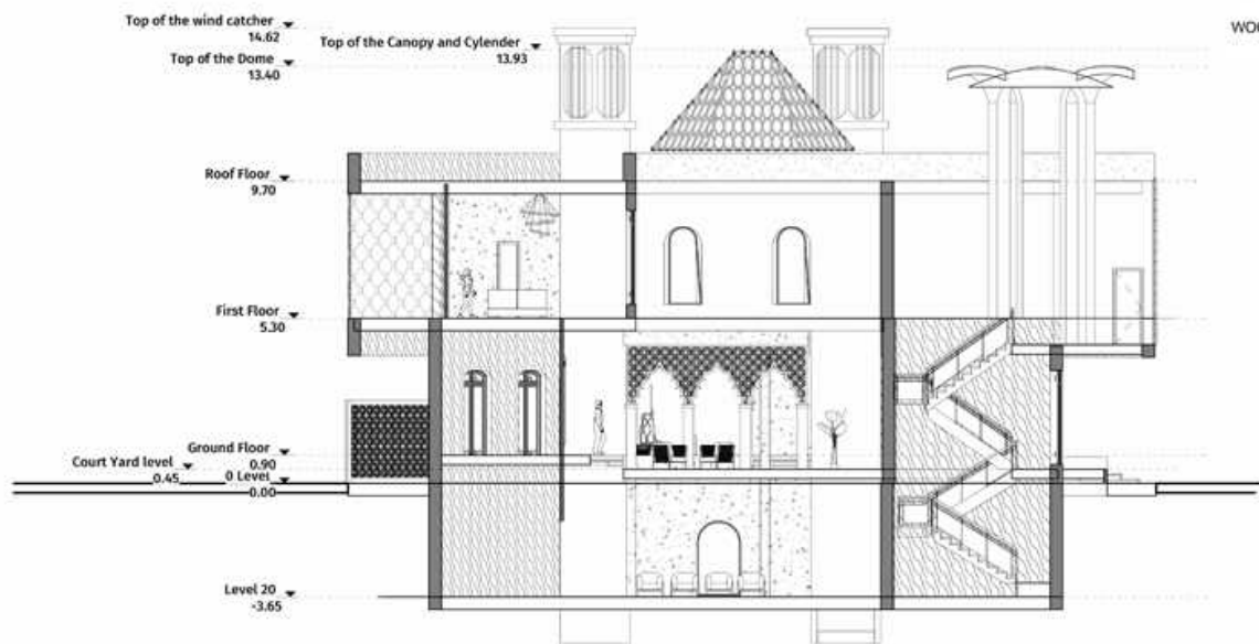
1 Section B-B 1 : 100
