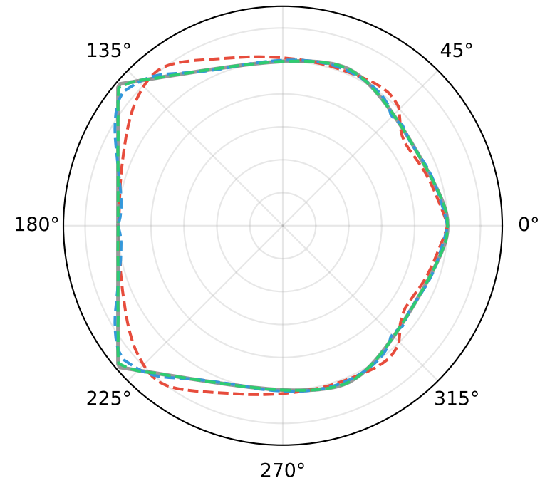
ID: 219 | Developable mot MSE(10): 9.6e-07 90°
