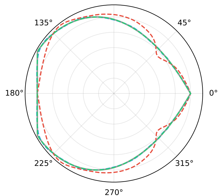
ID: 224 | Luna Rossa (Ita) MSE(10): 1.6e-07
