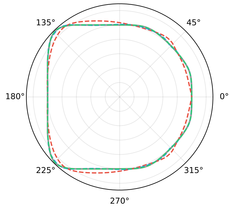
ID: 272 | 26 meter tug MSE(10): 2.4e-07 90° — Truth - - N=3 - - N=10 - - N=40
