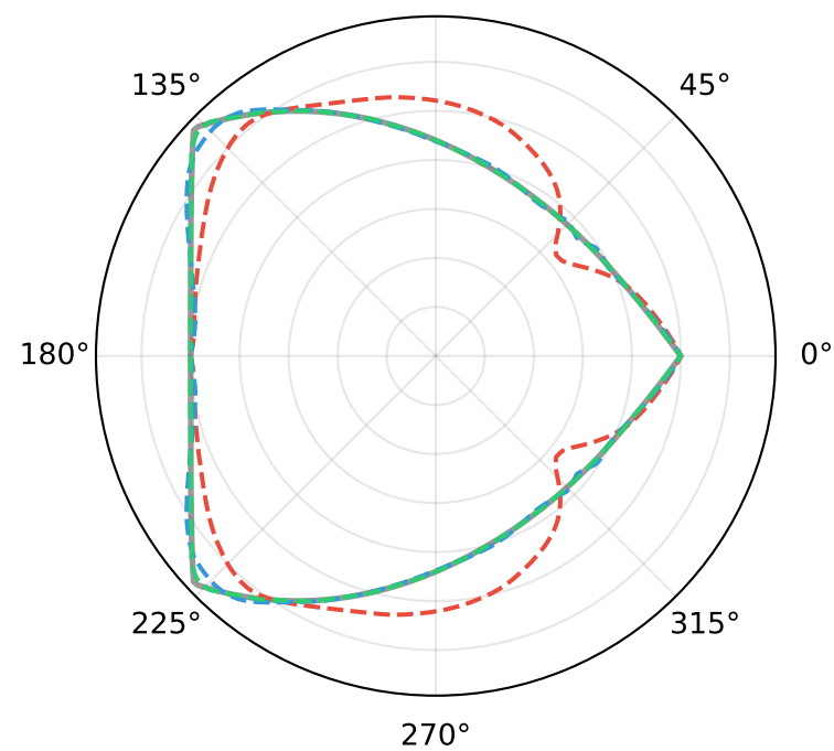
ID: 276 | 11m hull JMN MSE(10): 1.0e-06 90°
