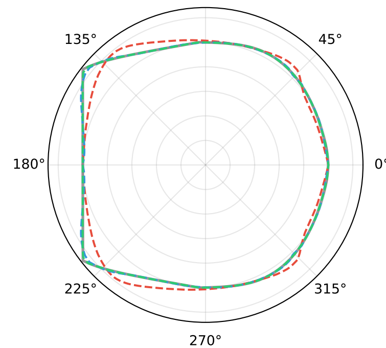
ID: 3 | Pegasus MSE(10): 3.3e-07 90°
