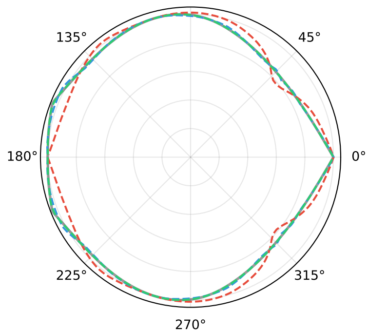
ID: 59 | s spant 1600 MSE(10): 3.4e-07 90°
