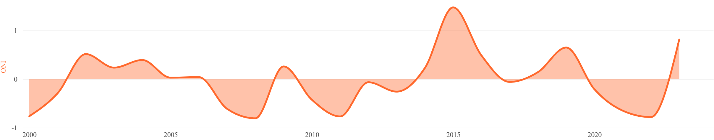
Índice ONI promedio por año (> 0,5 = El Niño, < -0,5 = La Niña)
