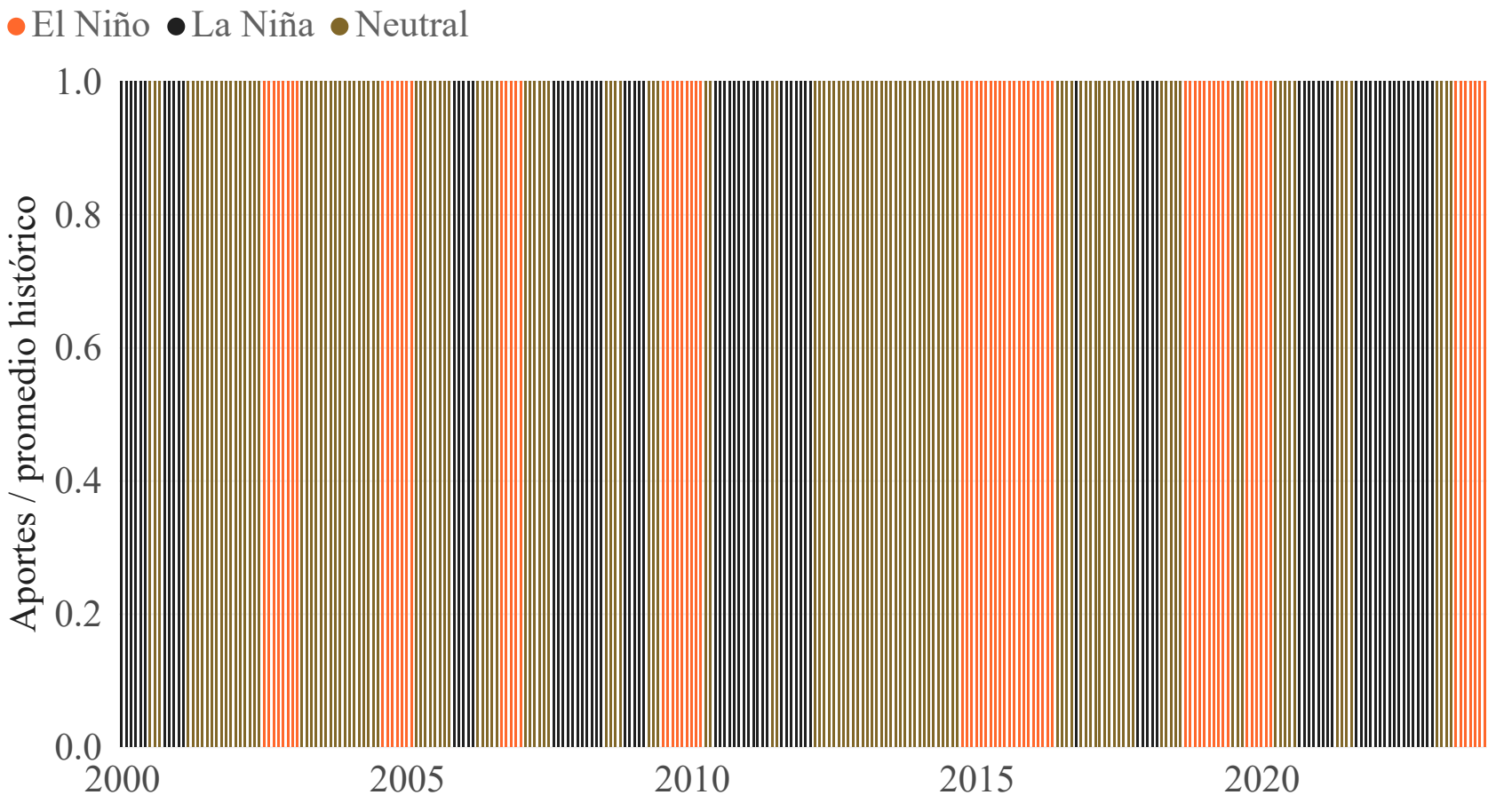
Aportes hídricos vs su promedio histórico, por fase ENSO
