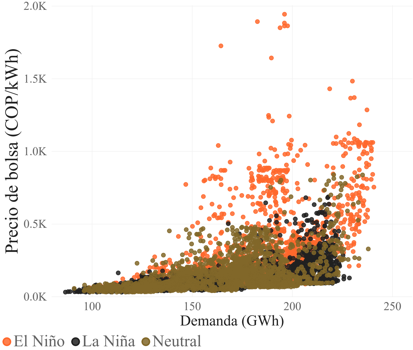
Demanda diaria vs precio, por fase ENSO
