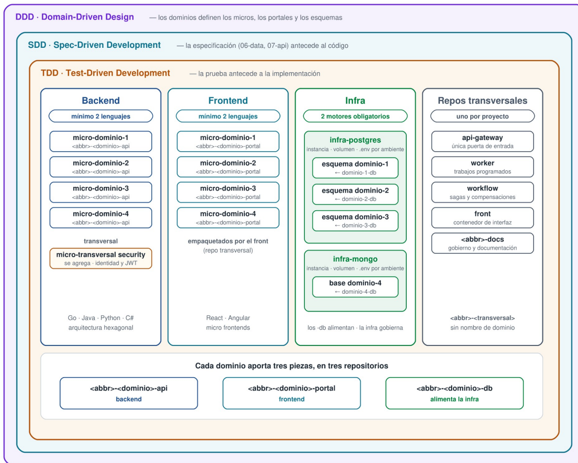
Figura 1. Infraestructura completa del proyecto: DDD, SDD y TDD envuelven todo el código.
