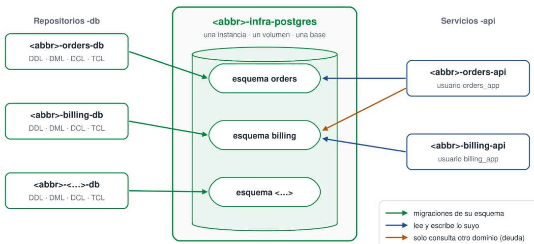
Figura 3. Una base, varios dueños: cada -db migra su esquema y cada servicio se conecta con su propio usuario.
