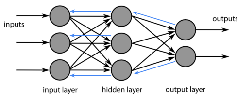
Figura 2.8: Arquitectura de red neuronal con conexiones feedforward e incluyendo conexiones top-down resaltadas en azul.
