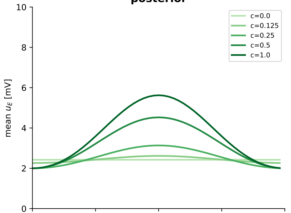
posterior
