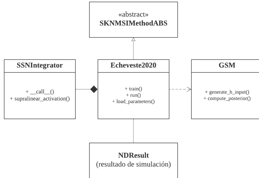
Figura 5.1: Diagrama de clases UML simplificado de la implementación del modelo de Echeveste. Para una versión detallada, véase la Figura A.2.
