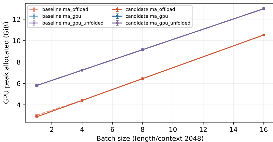
Prefill
