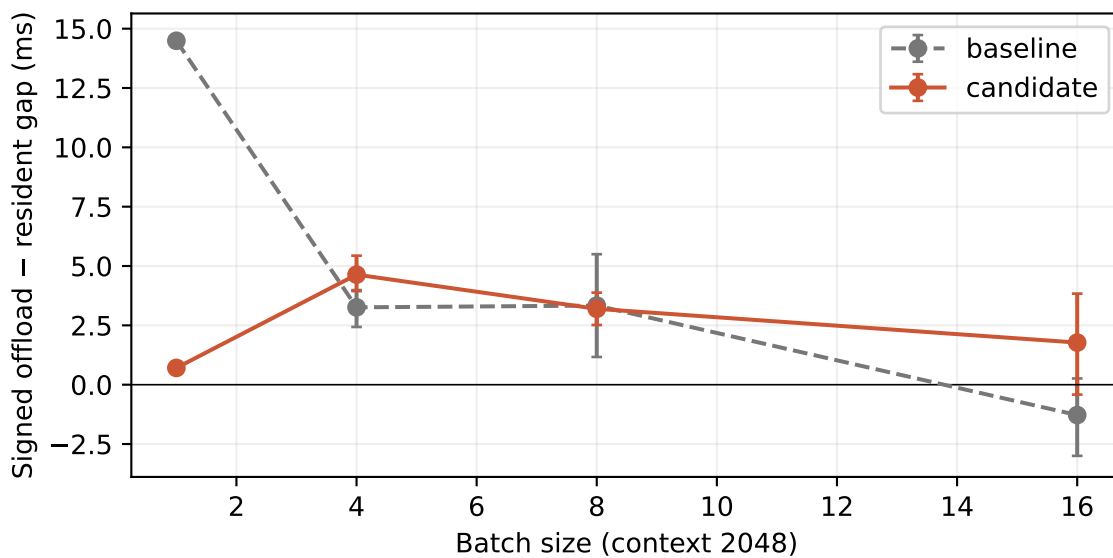
Prefill
