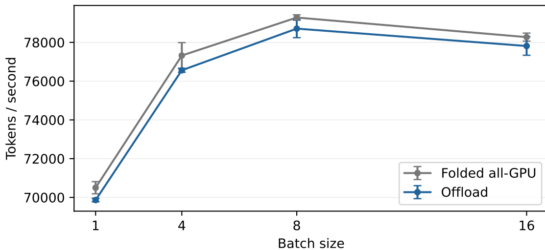
Decode · context 2048
